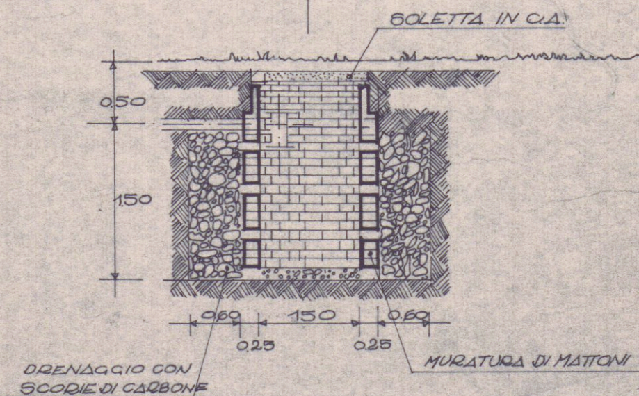
SEZIONE
