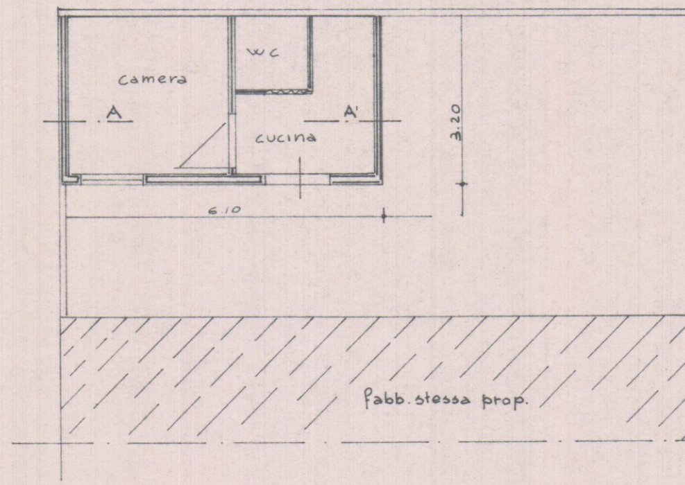
PIANTA
