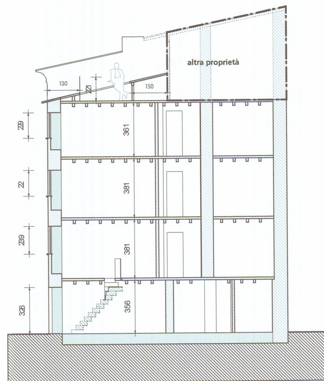
6 sezione scala 1: 100
