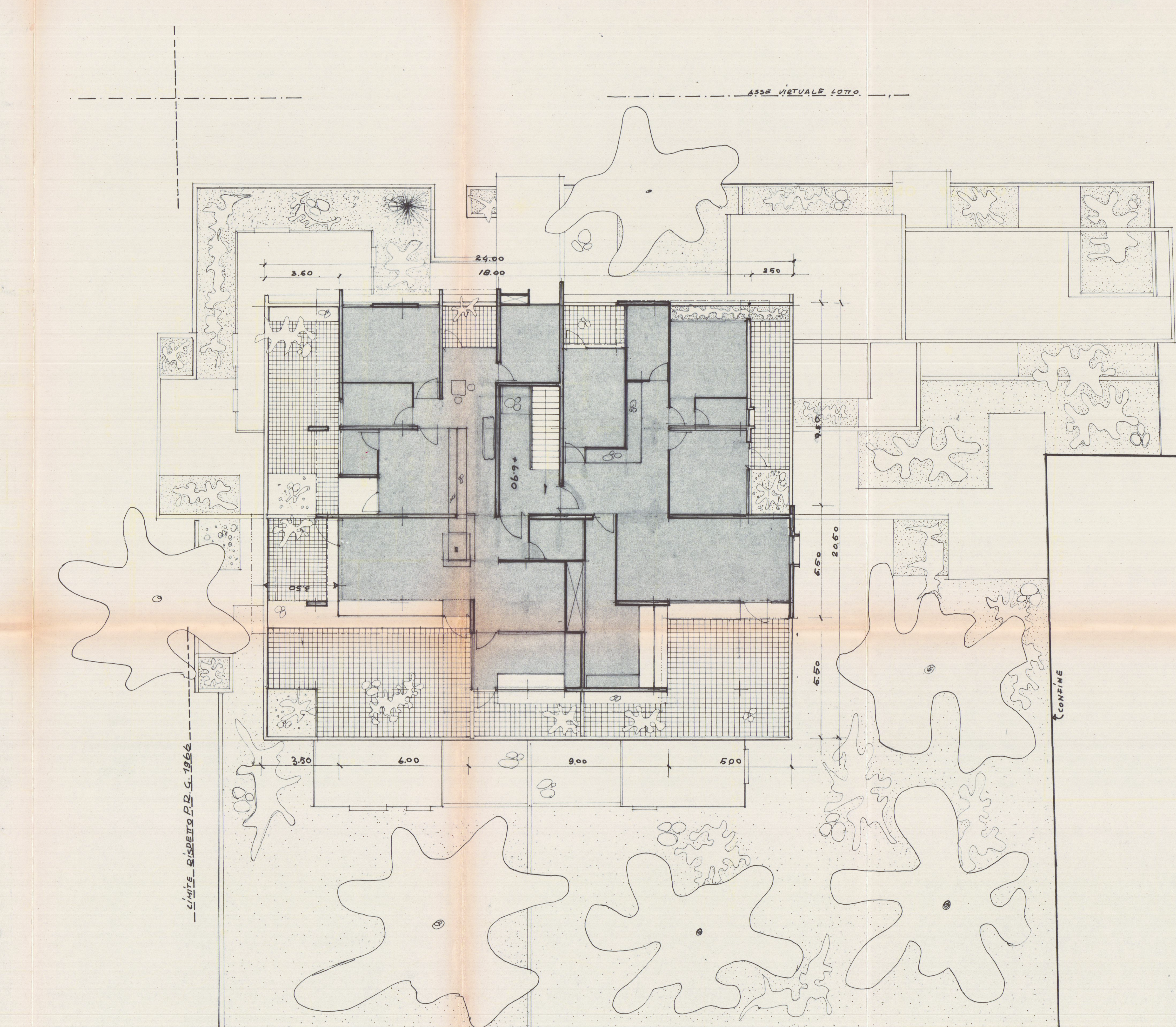
PIANTA PIANO ATTICO mq. 340
