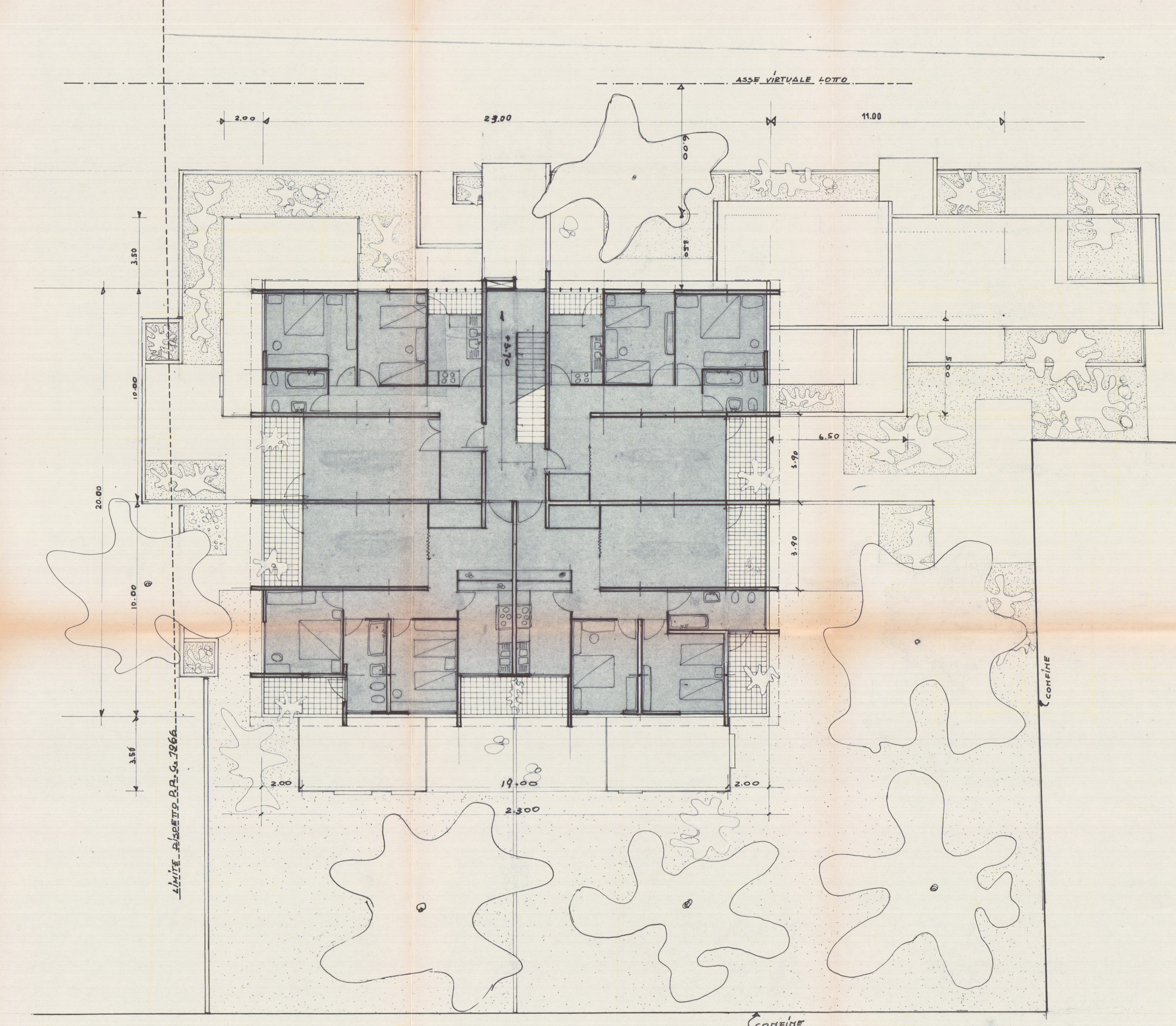
PIANTA PRIMO PIANO mq. 397
