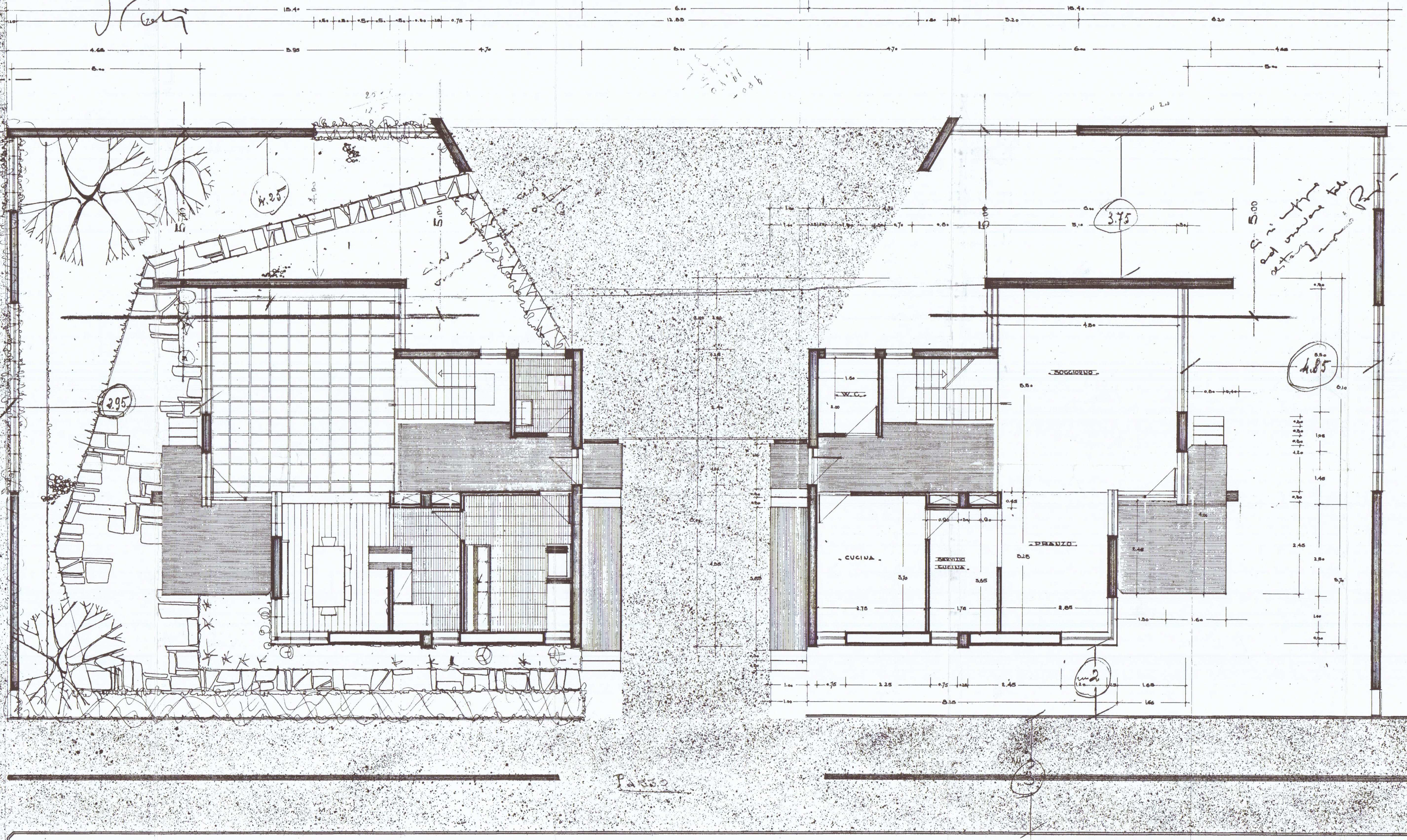
PIANTA DEL PIANO TERRA ED ARREDAMENTO GIARDINO - SCALA 1:50 -
