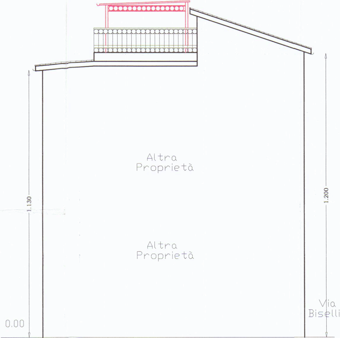
PROSPETTO NORD - OVEST
