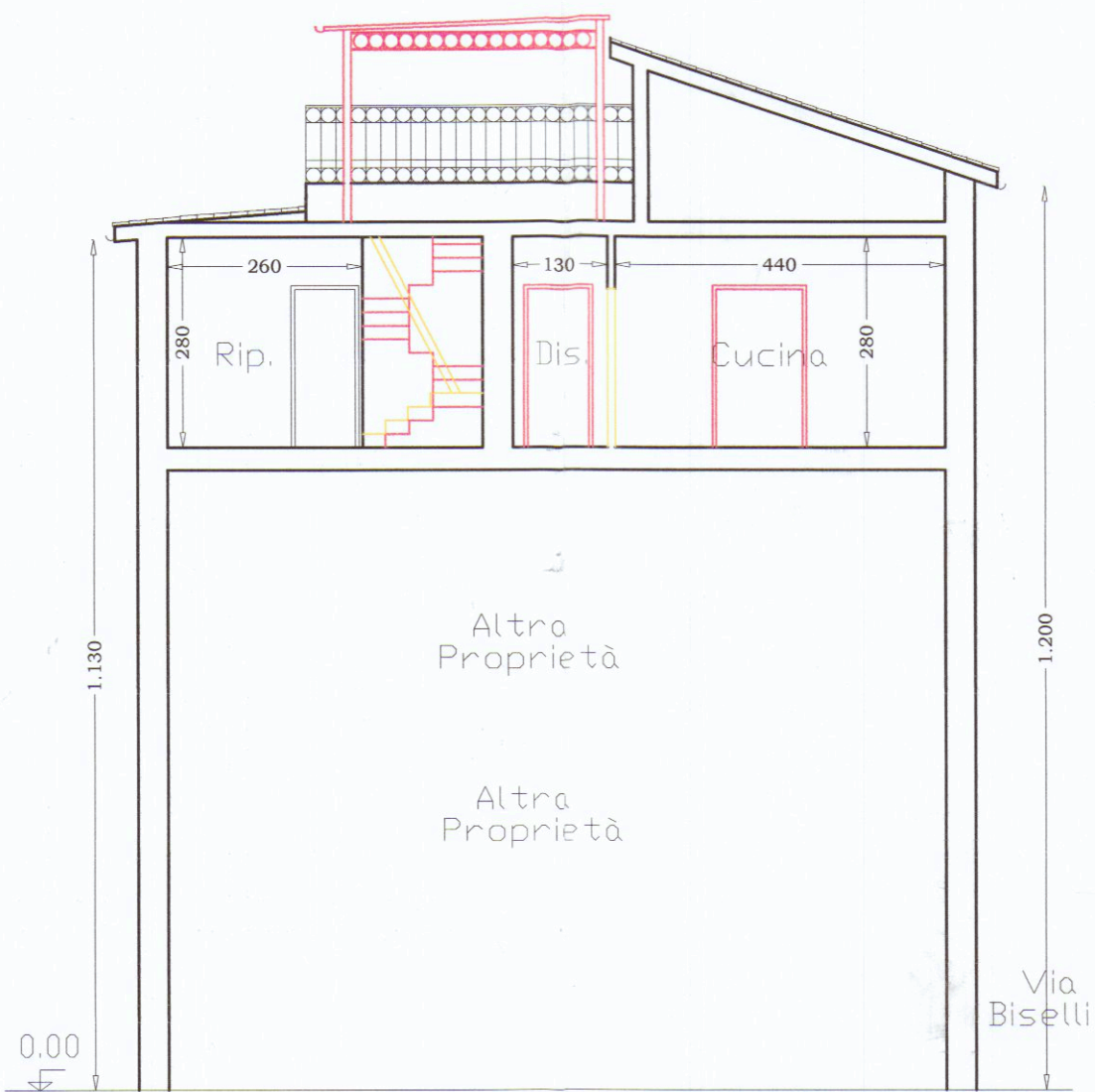
Sezione A-A'
