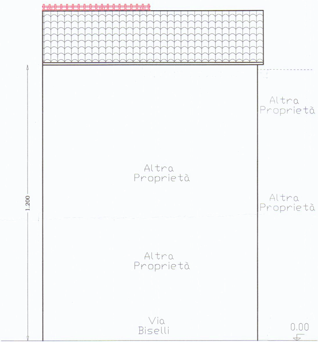
PROSPETTO SUD - OVEST
