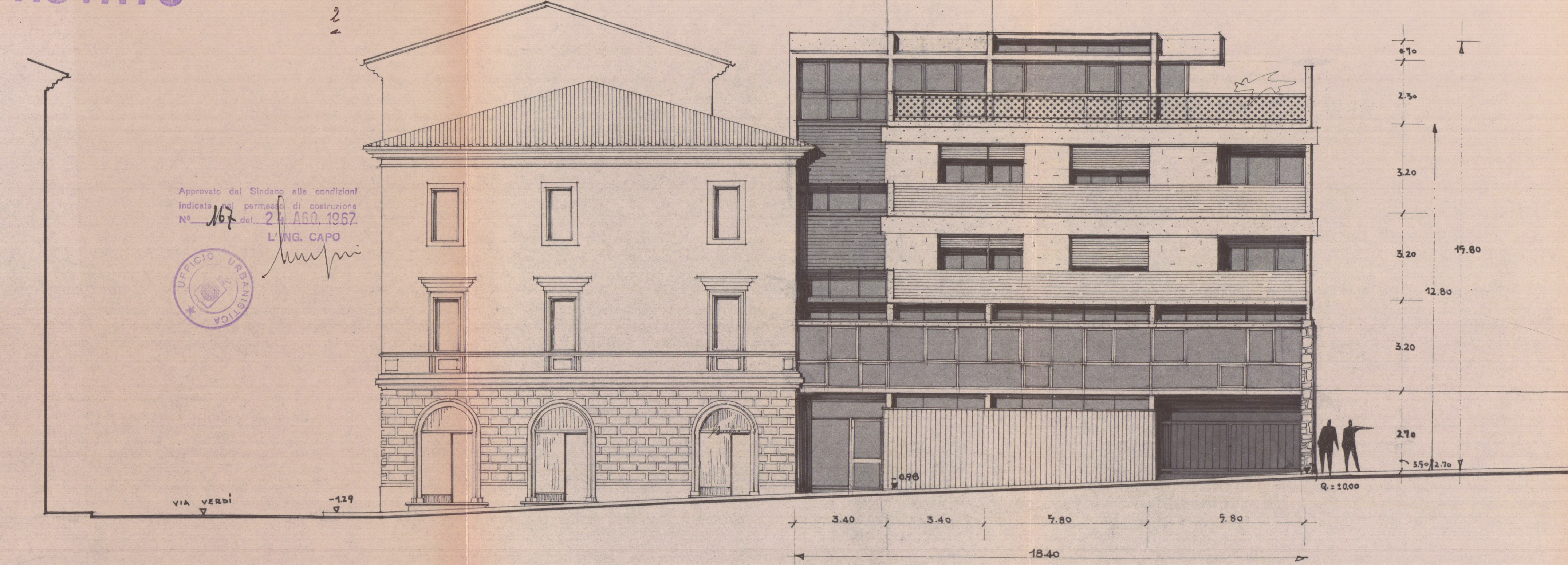
- RAPP. 1:100 - - PROSPETTO SU VIA SOLFERINO
