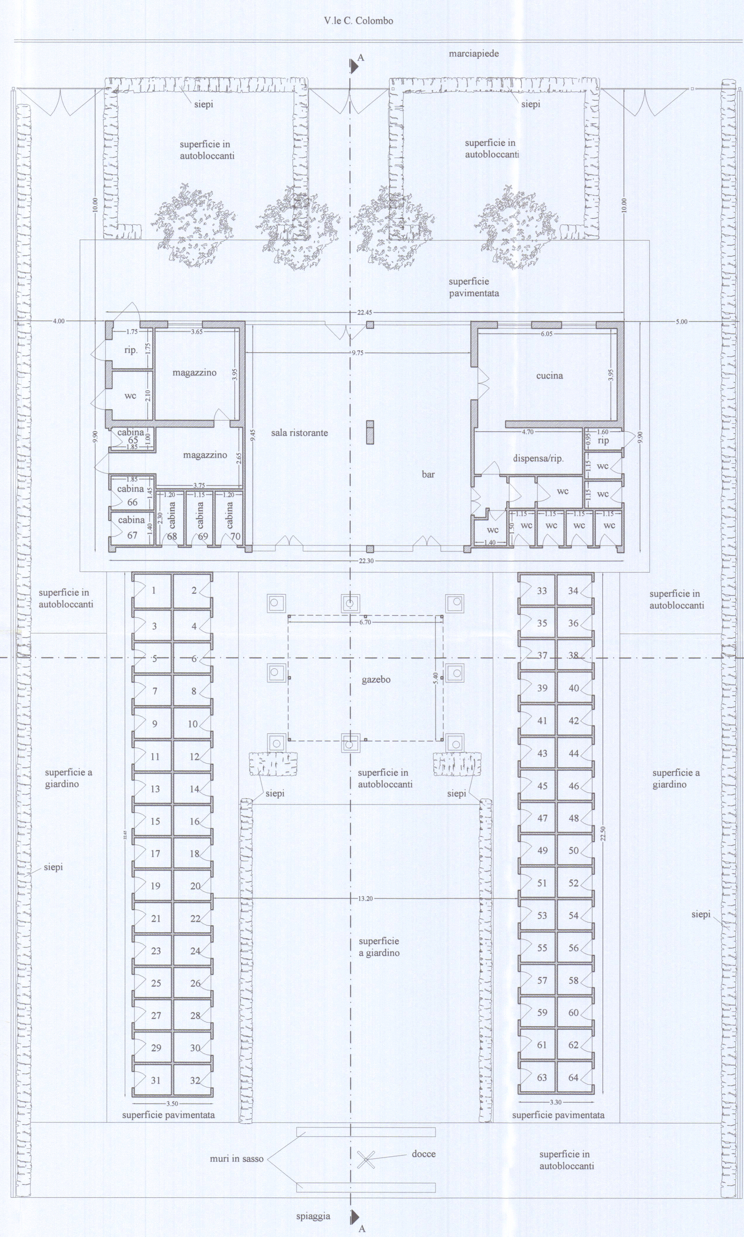
PIANTA PIANO TERRA
