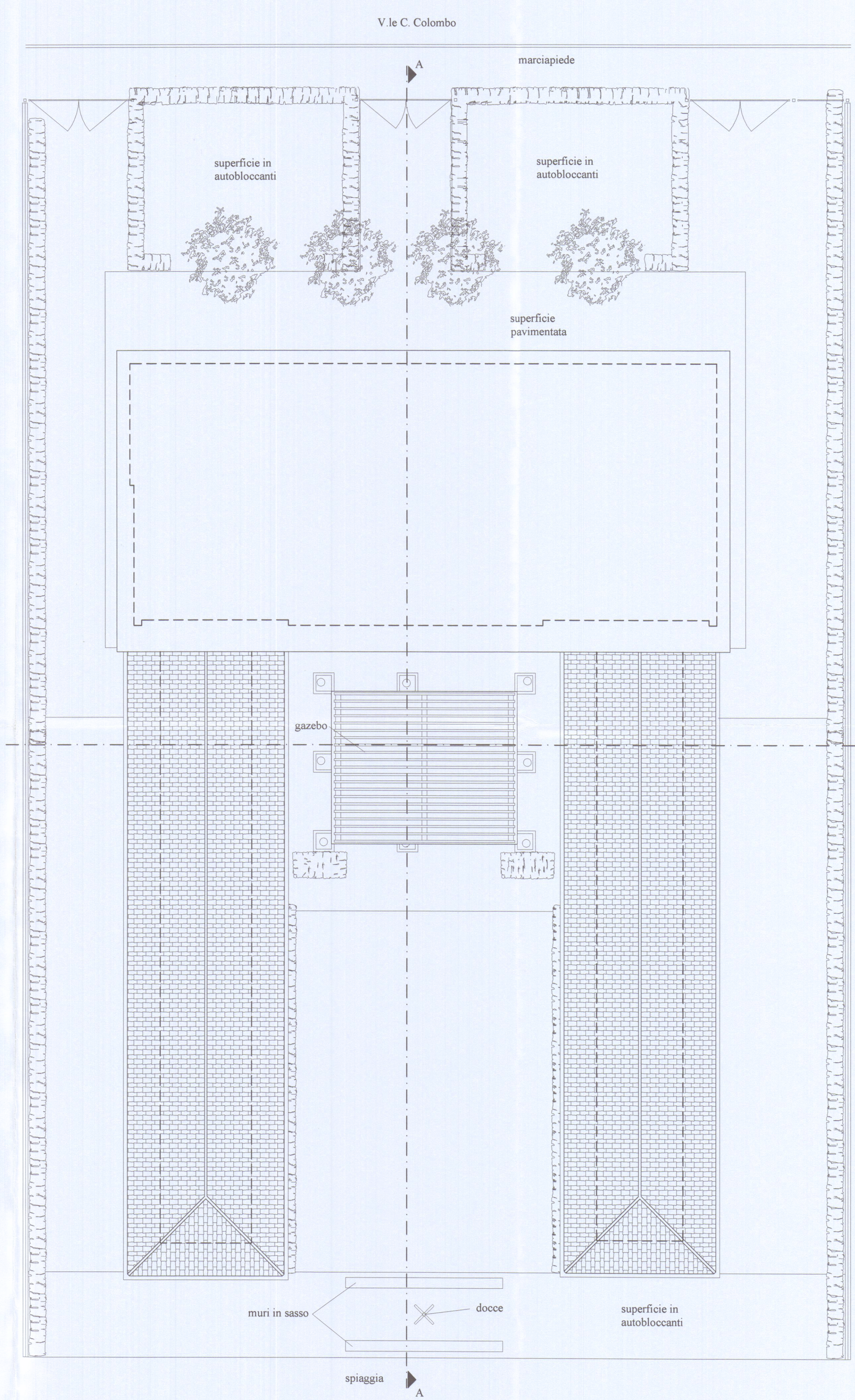
PIANTA COPERTURA
