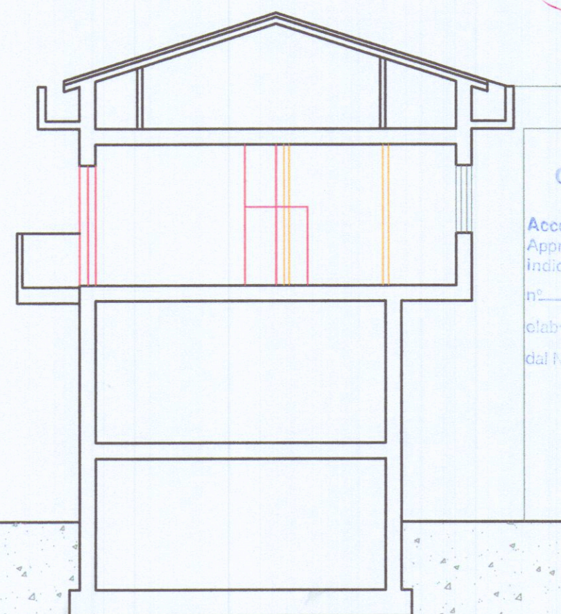
Sezione A-A'
