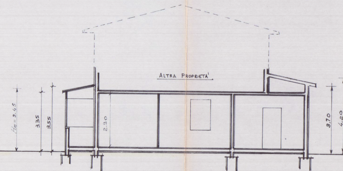
SEZIONE A-A
