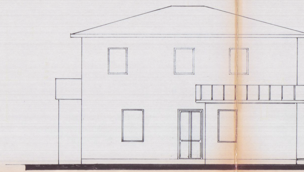
PROSPETTO OVEST
