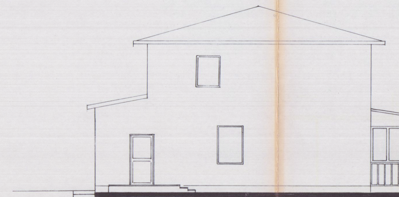
PROSPETTO SUD
