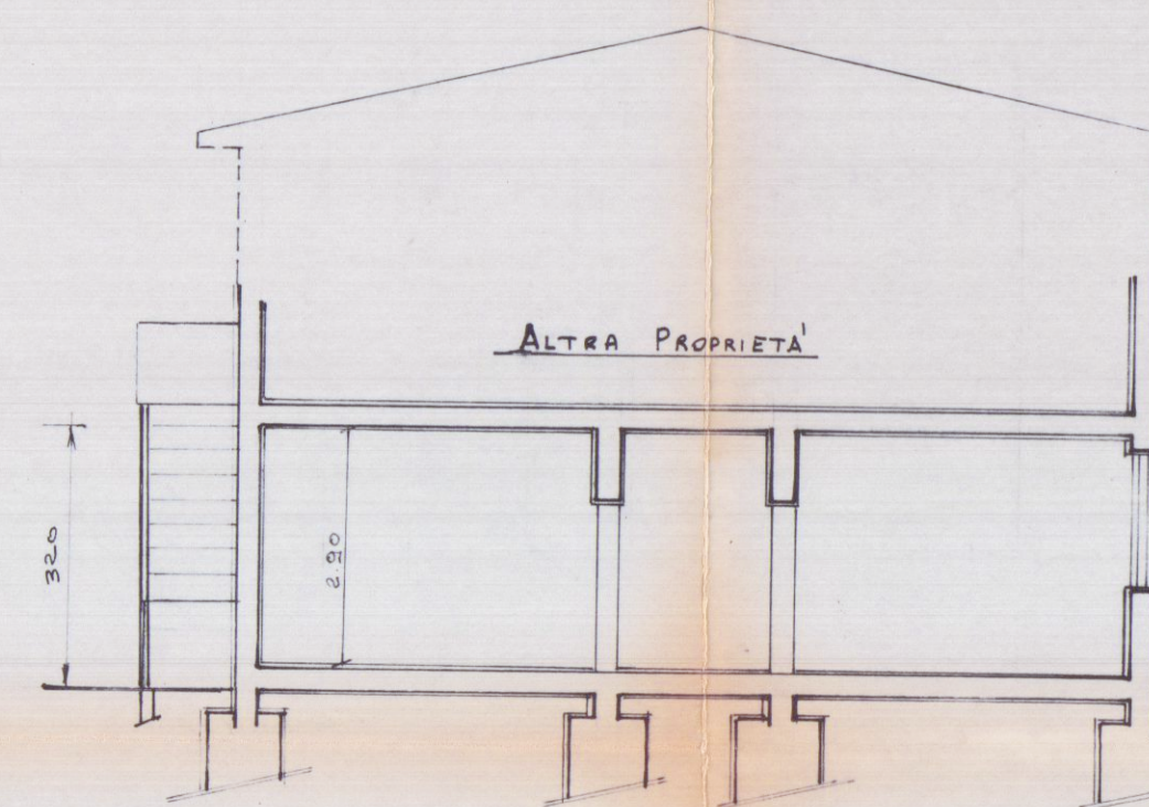
SEZIONE B-B
