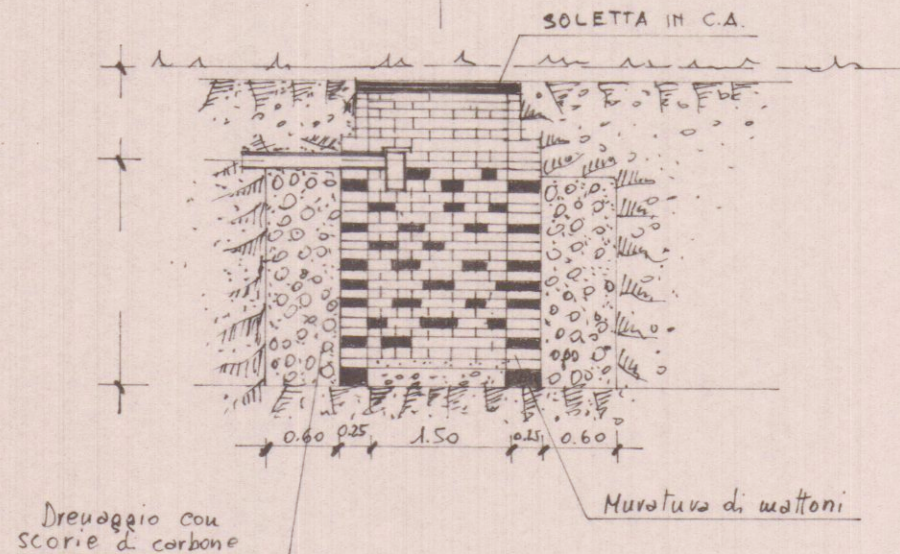
SEZIONE A-B
