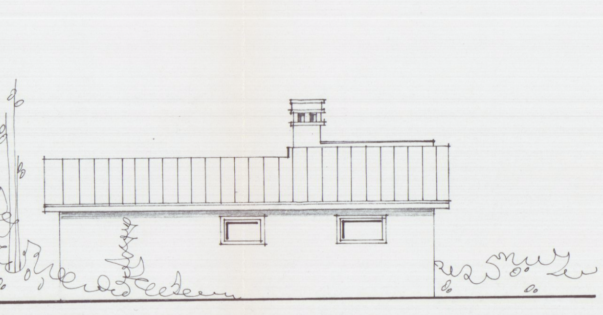
PROSPETTO EST
