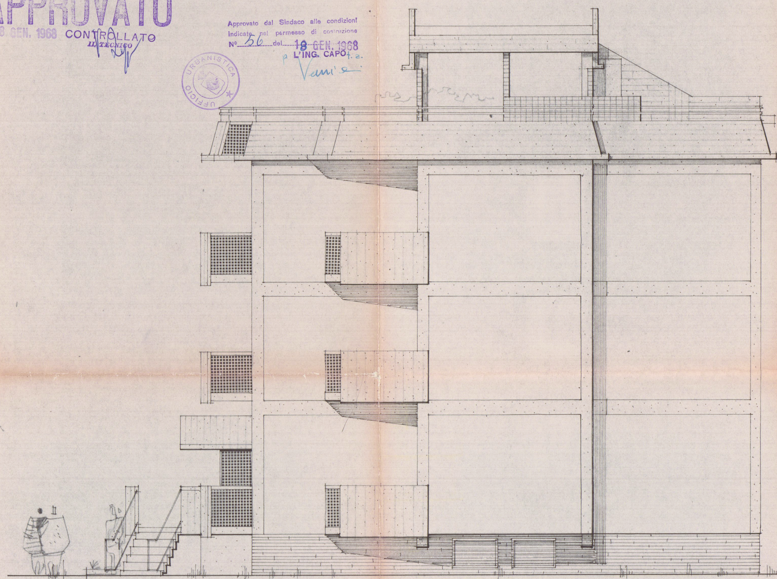
PROSPETTO EST
