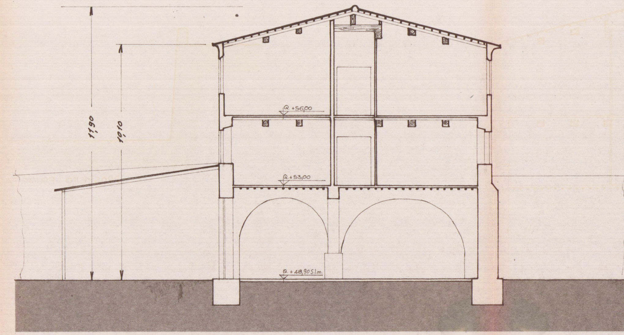
SEZIONE TRASVERSALE ESISTENTE a-b
