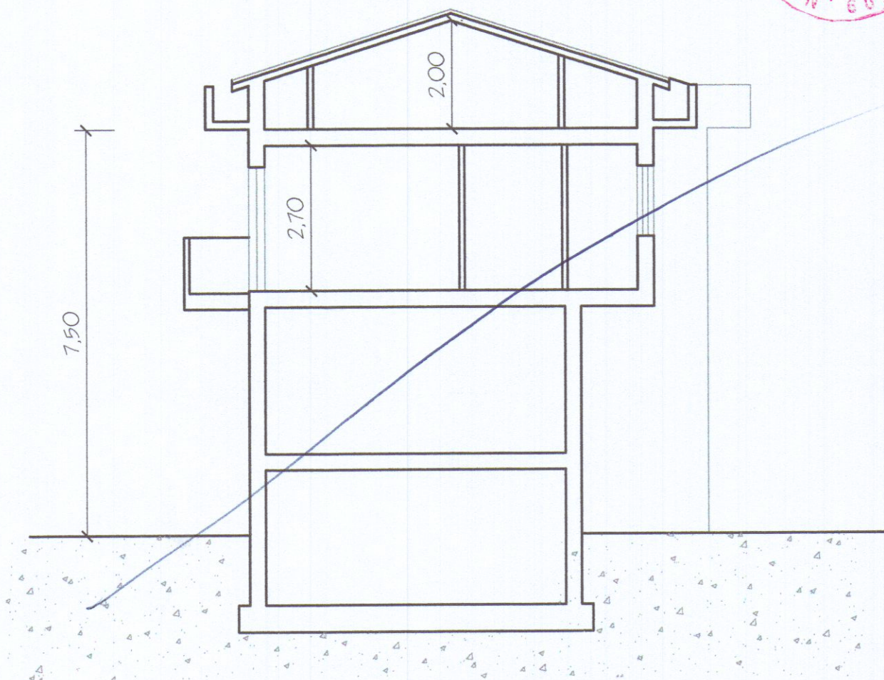
Sezione A-A'
