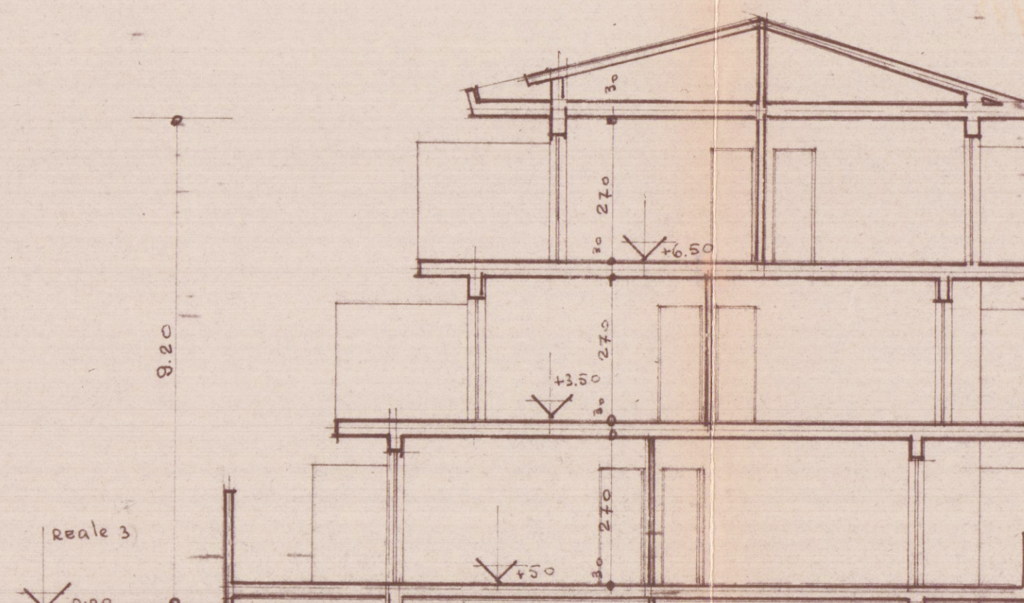
SEZIONE A-A
