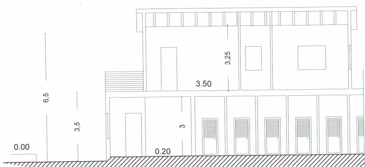
SEZIONE A-A
