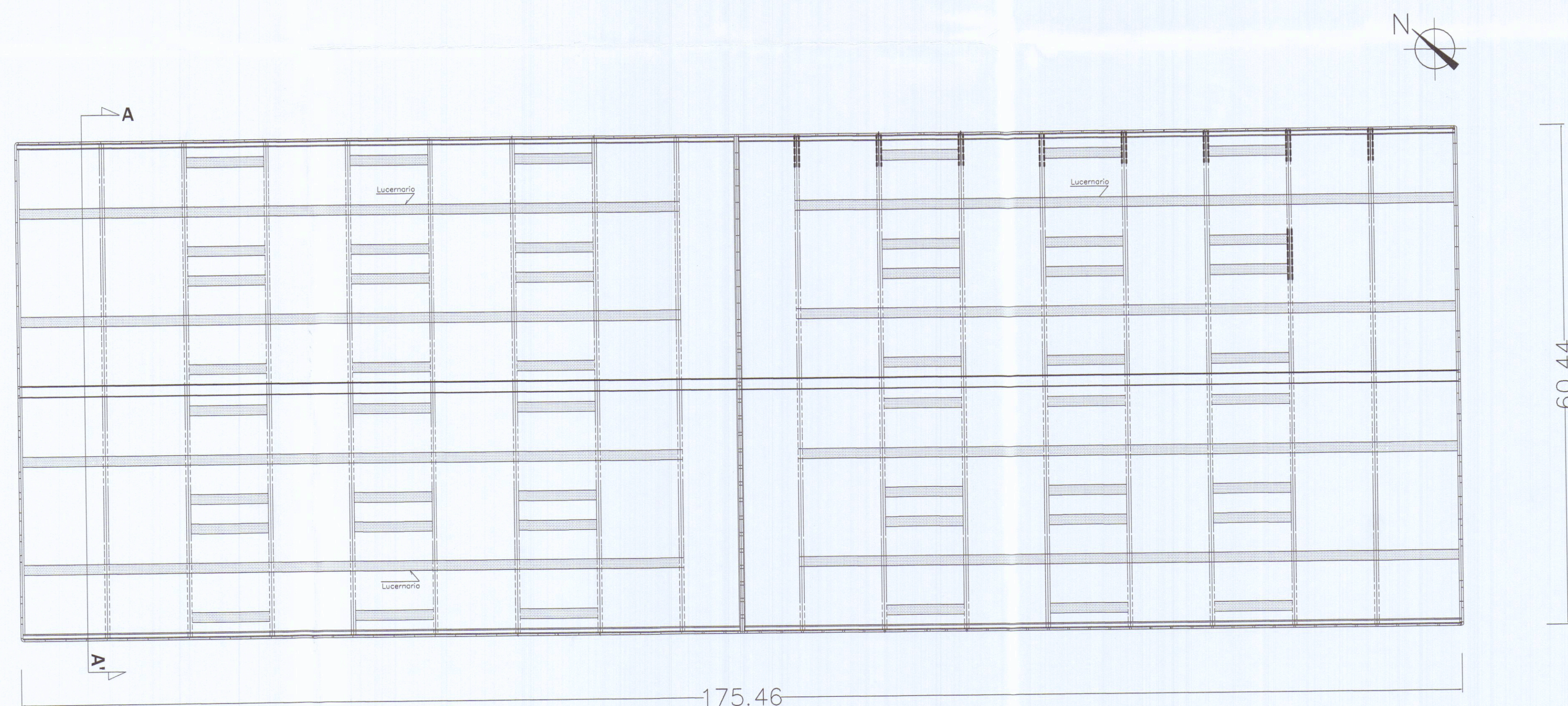
PIANTA COPERTURA MAGAZZINO
