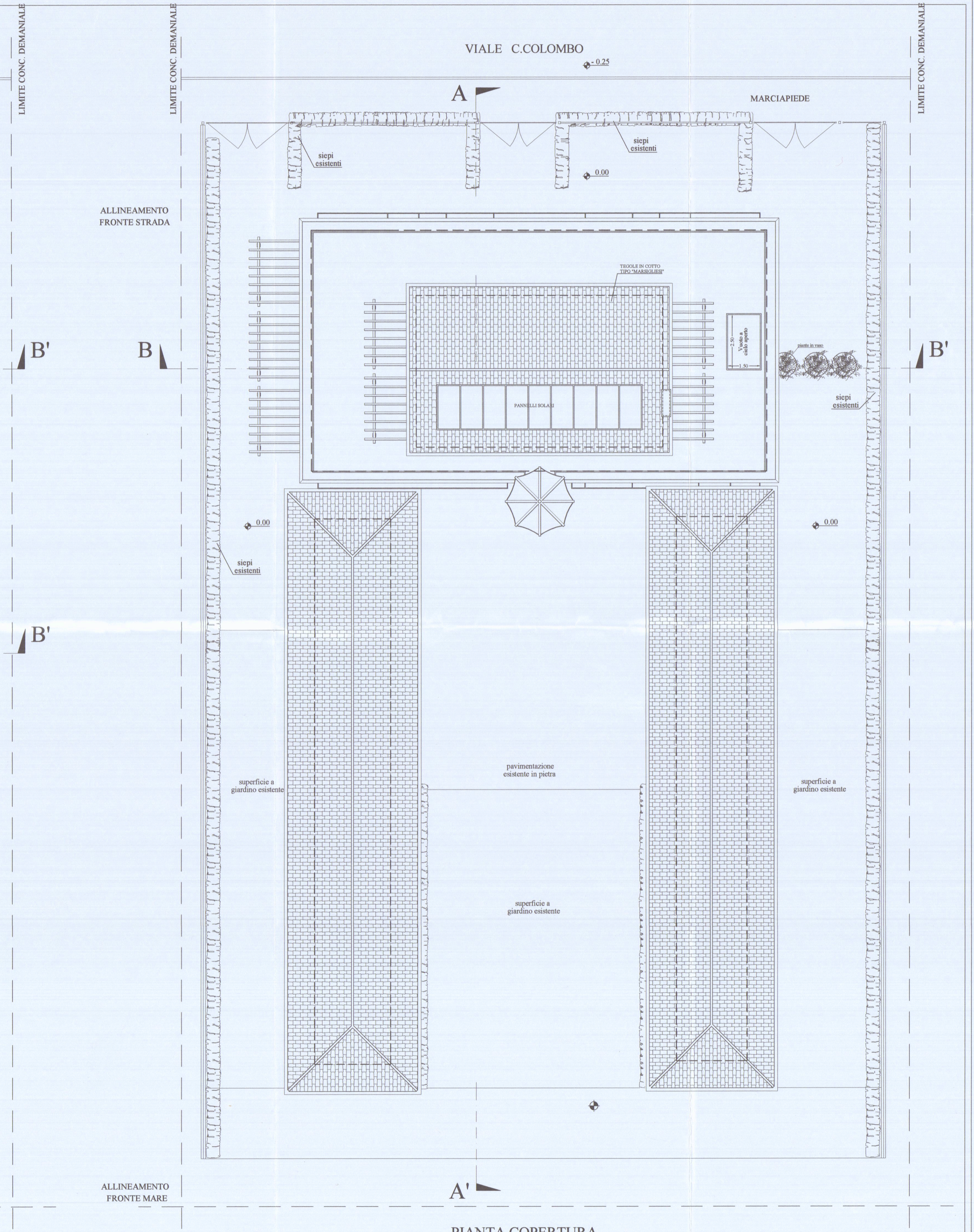
PIANTA COPERTURA
