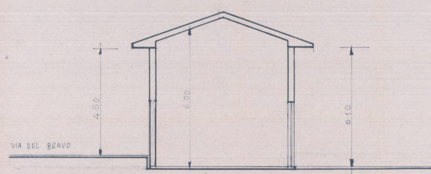
SEZIONE A-A
