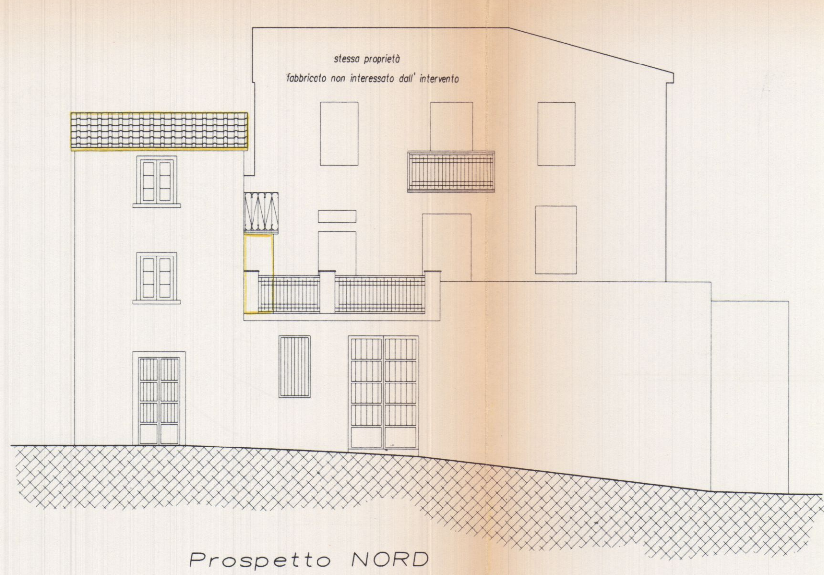
Prospetto NORD
