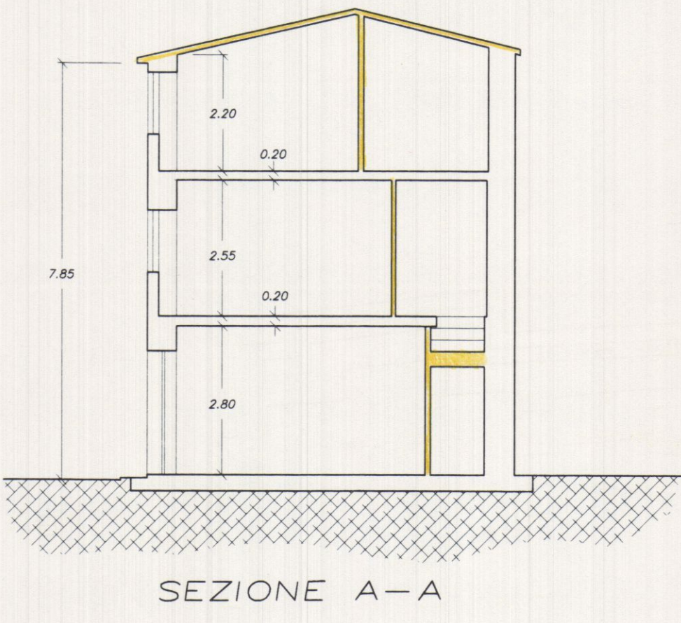
SEZIONE A-A
