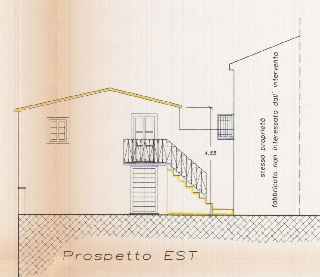
Prospetto EST
