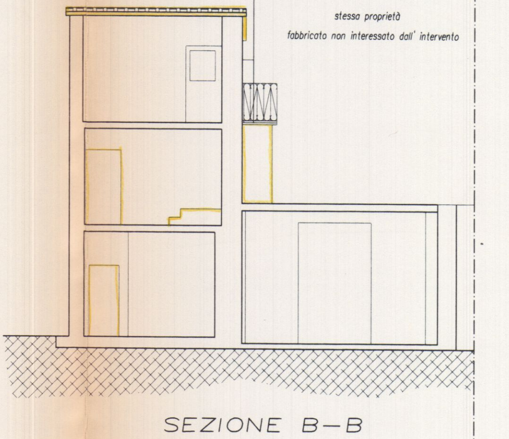
SEZIONE B-B
