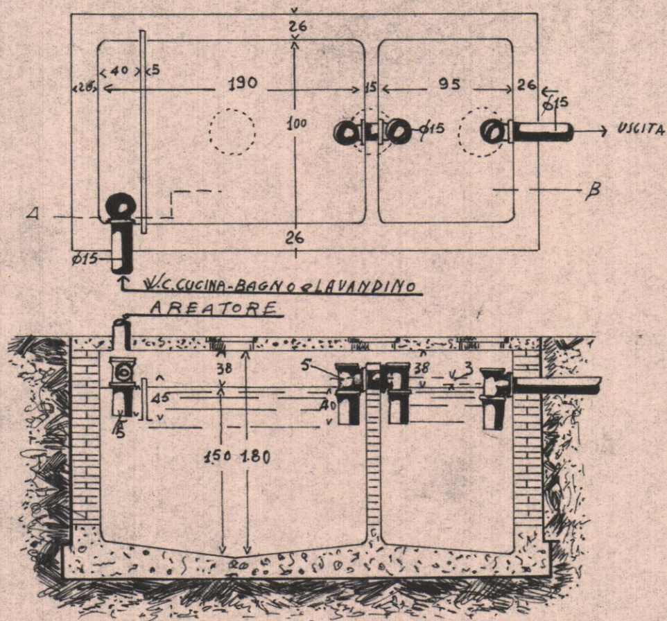
SEZIONE A-B
