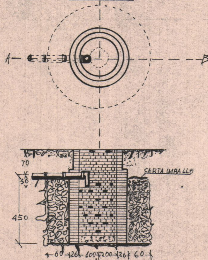
TIPO DI POZZETTO PERDENTE
