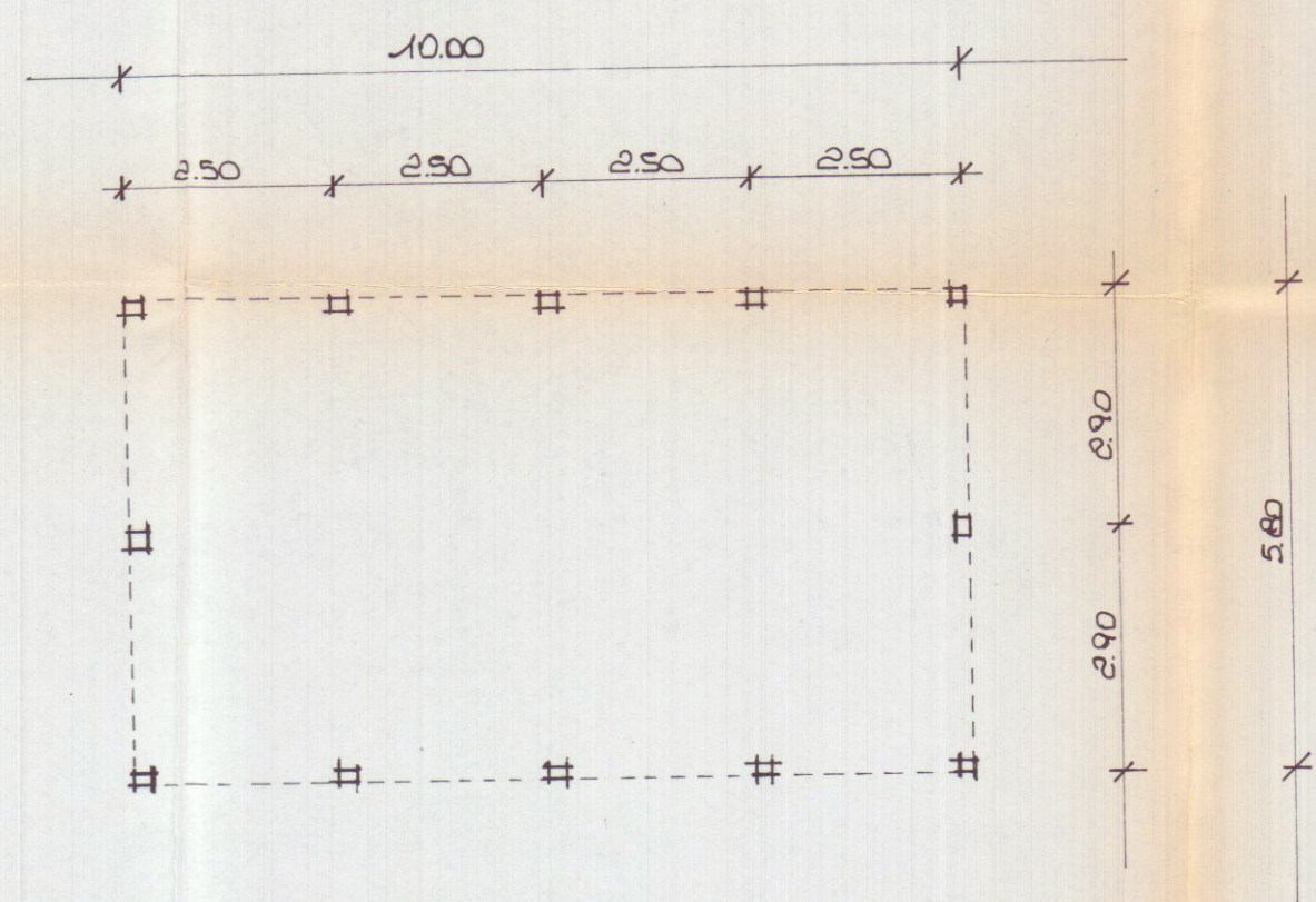
- Pianta Scala 1:100 -
