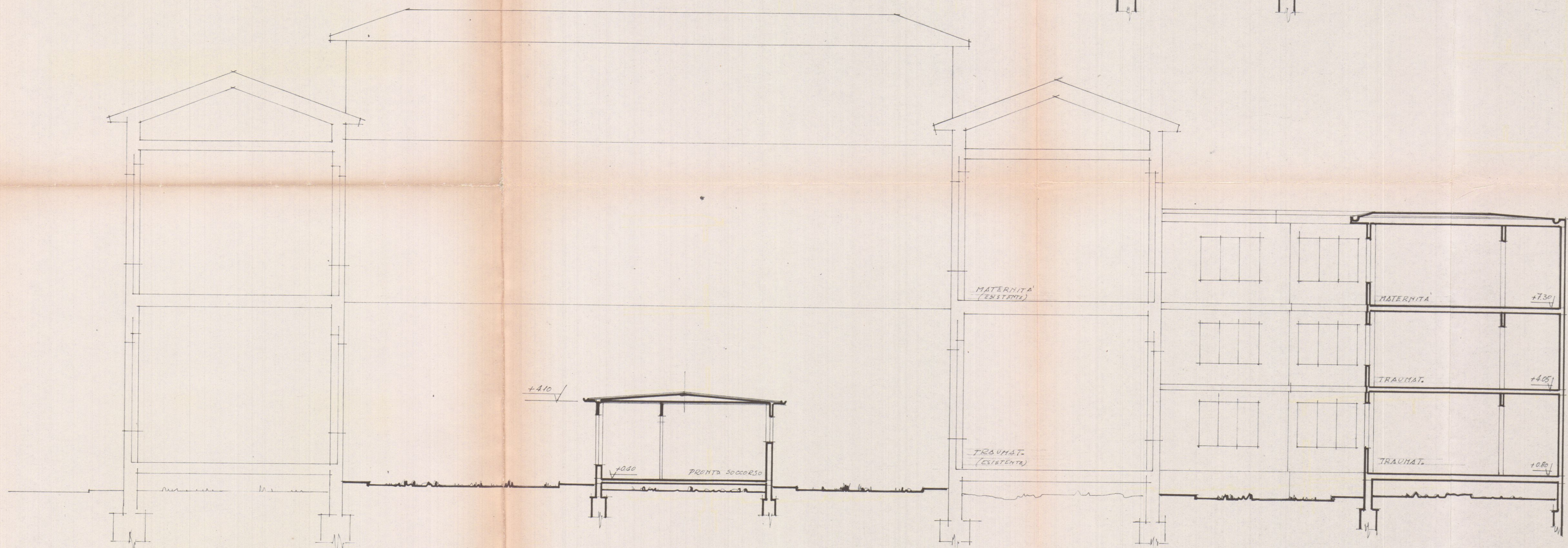
SEZIONE 1-1
