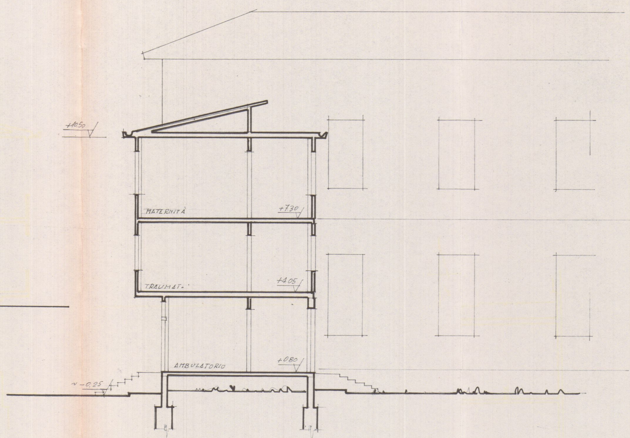
SEZIONE 2-2
