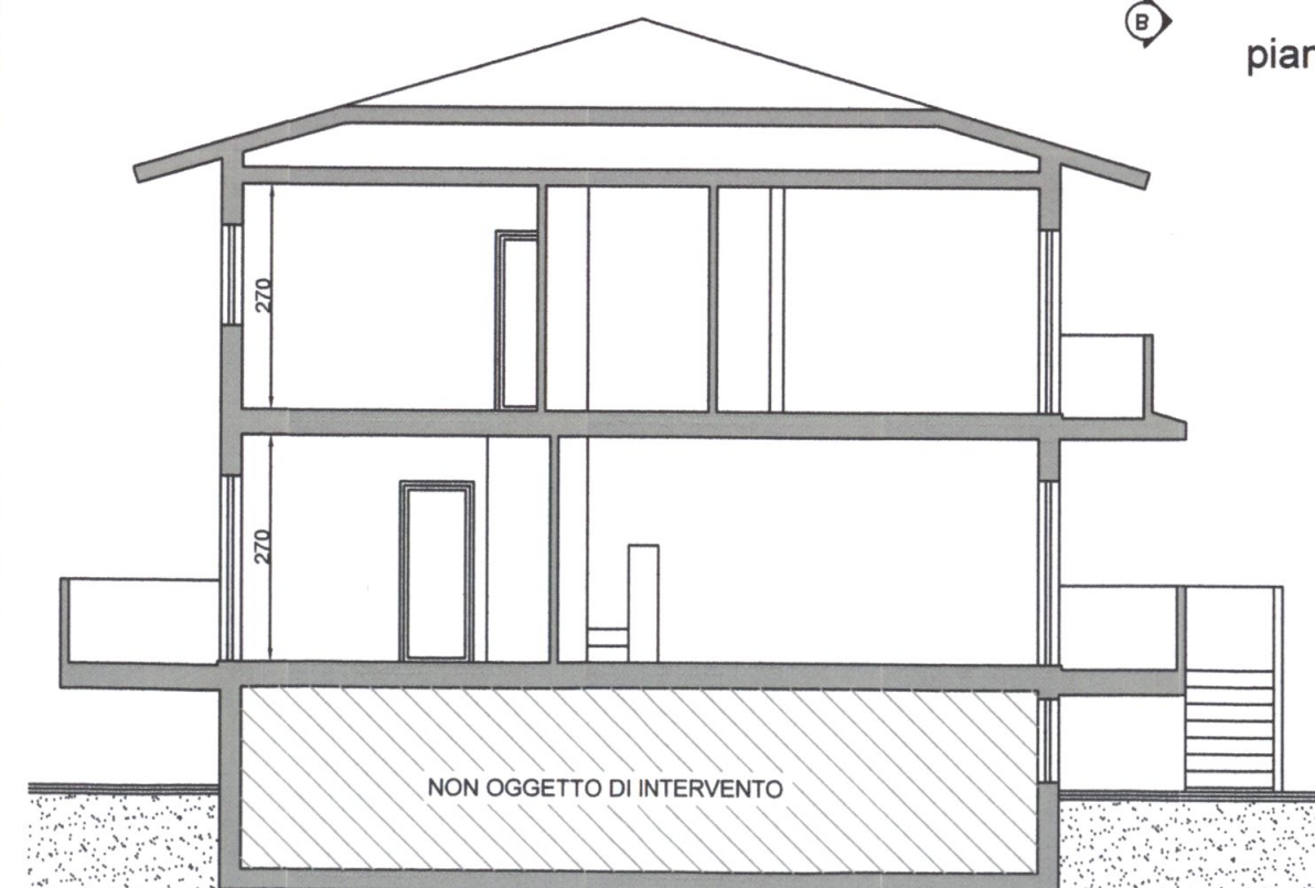
sezione B-B
