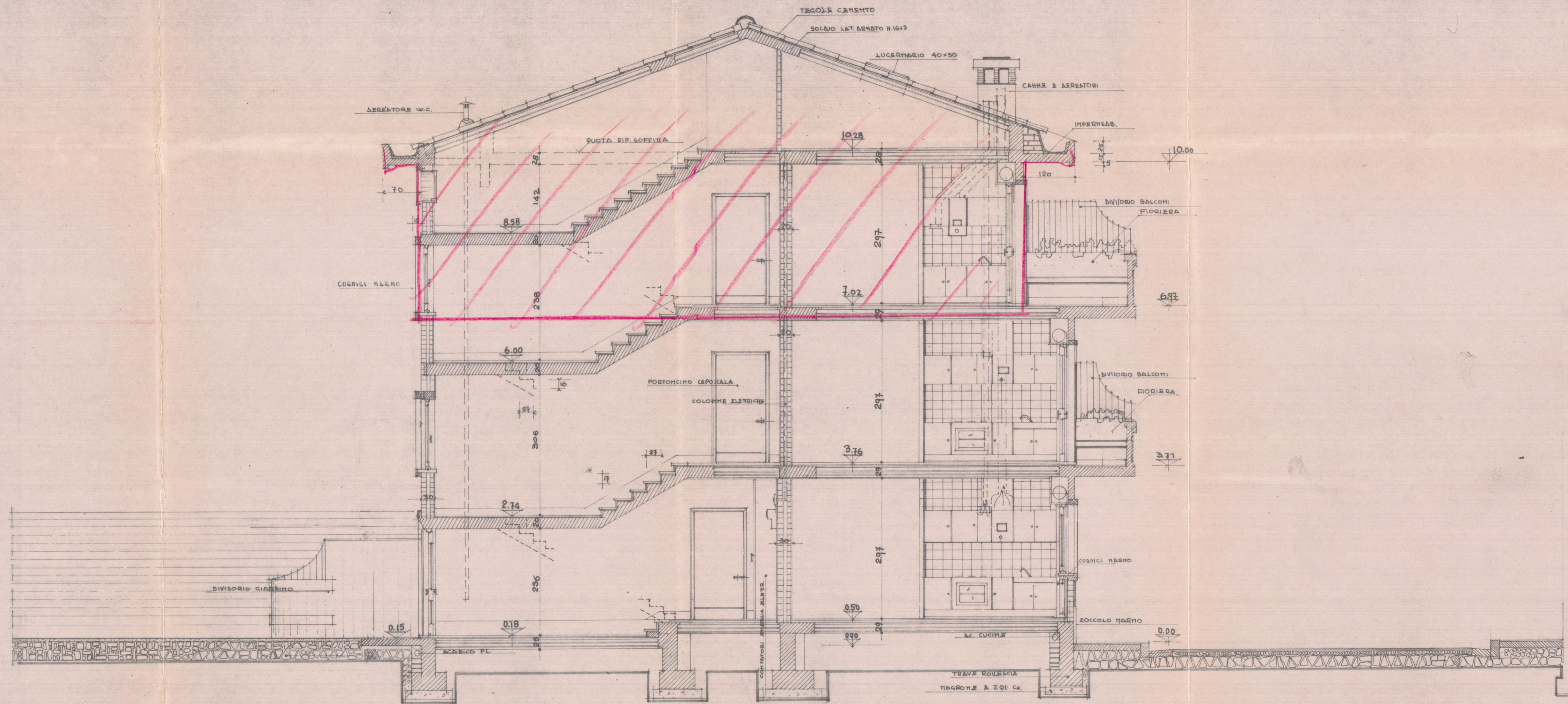
sezione A-B
