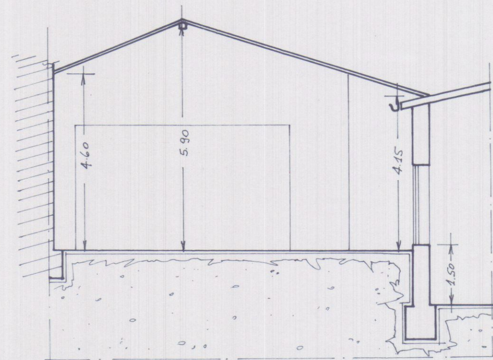
SEZIONE A-B - RADD. 1/100
