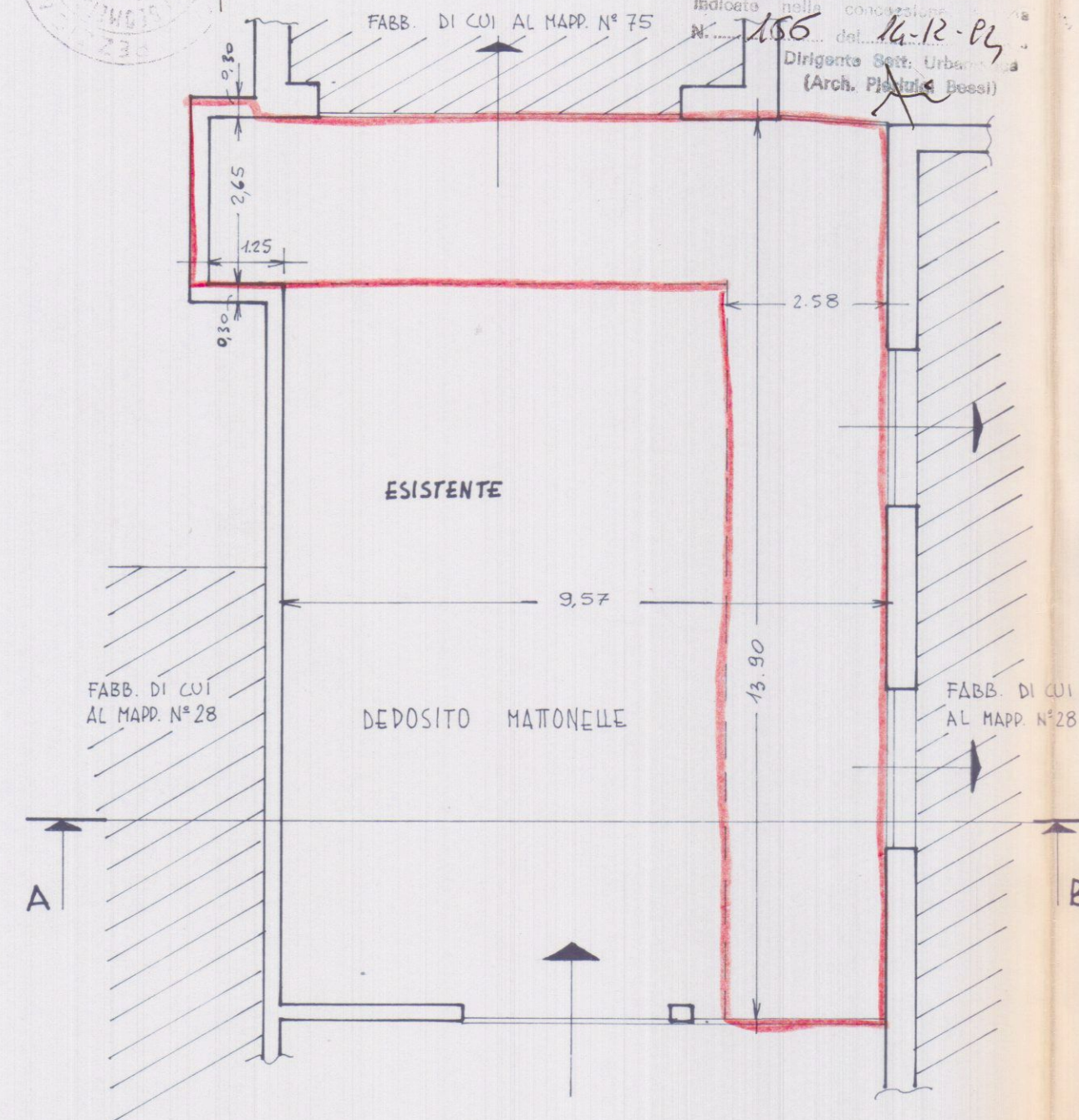
PIANTA - RADD. 1/100
