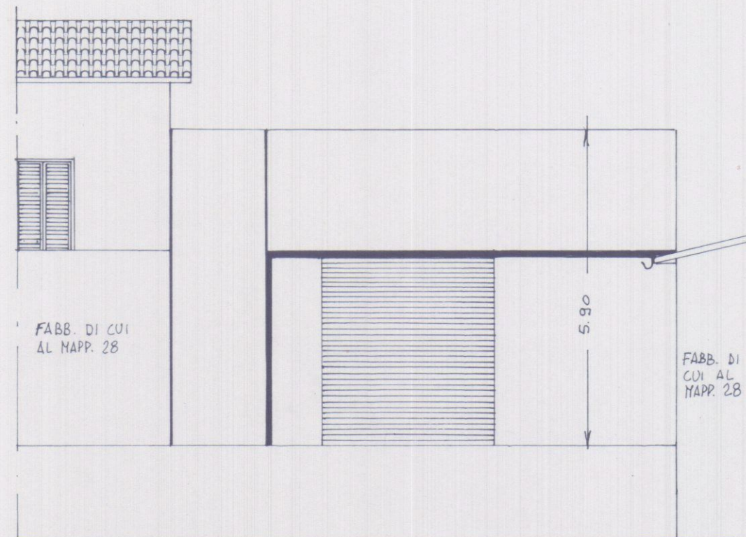
PROSPETTO VERSO DIAZZALE INTERNO RADD. 1/100
