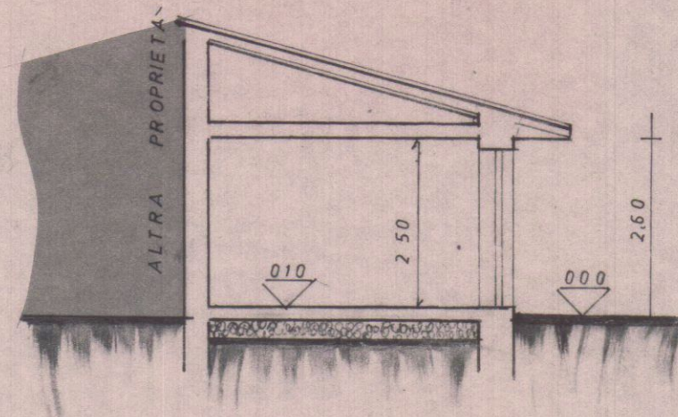
SEZIONE AA'
