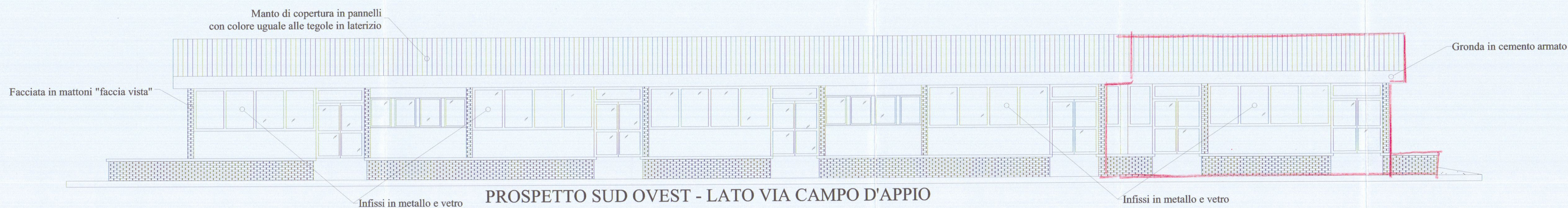
PROSPETTO SUD OVEST - LATO VIA CAMPO D'APPIO
