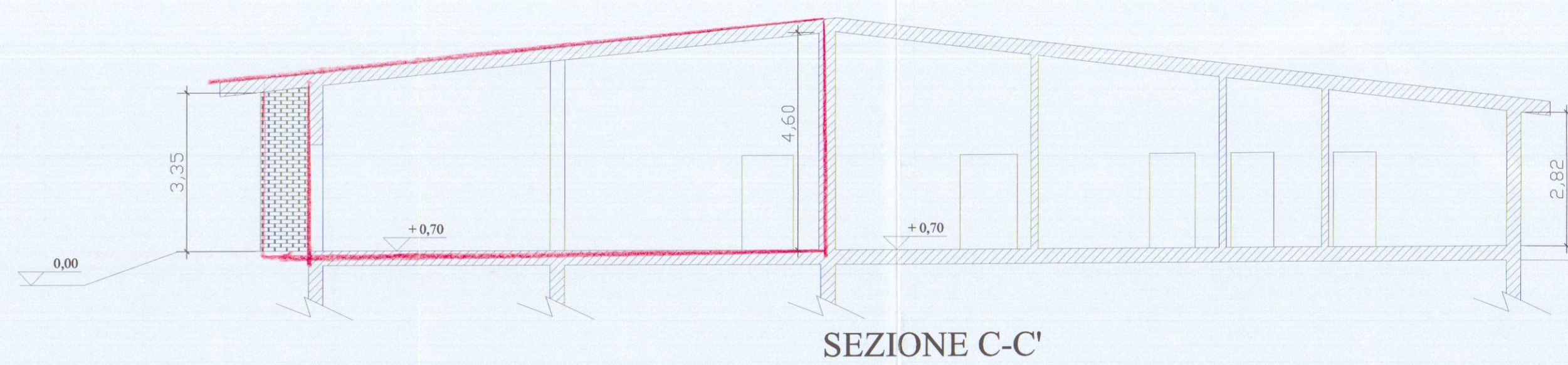
SEZIONE C-C'
