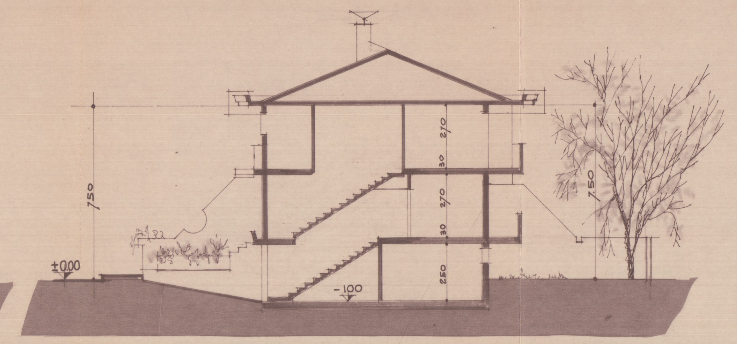
SEZIONE -B-
