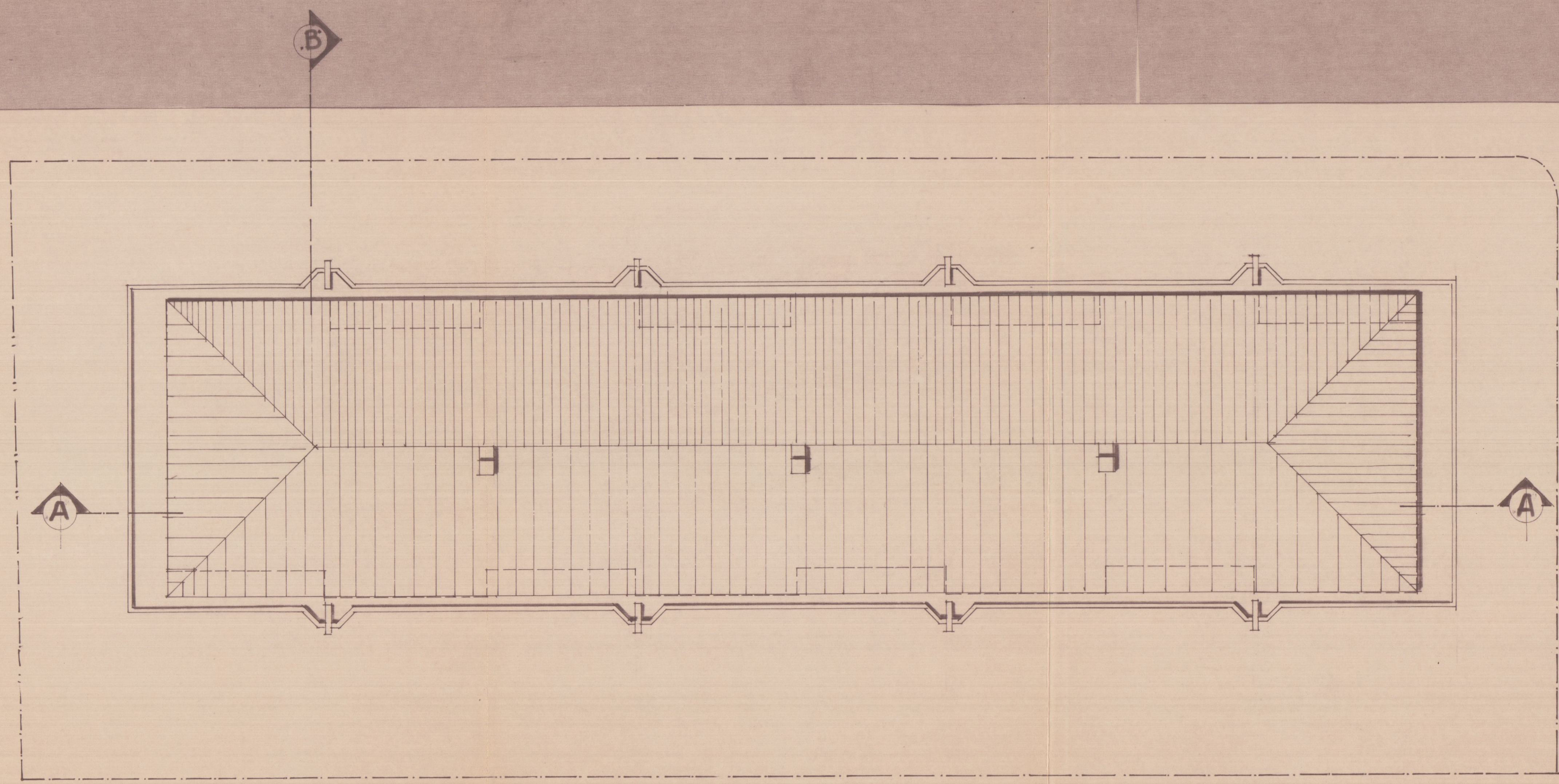
PIANTA COPERTURA
