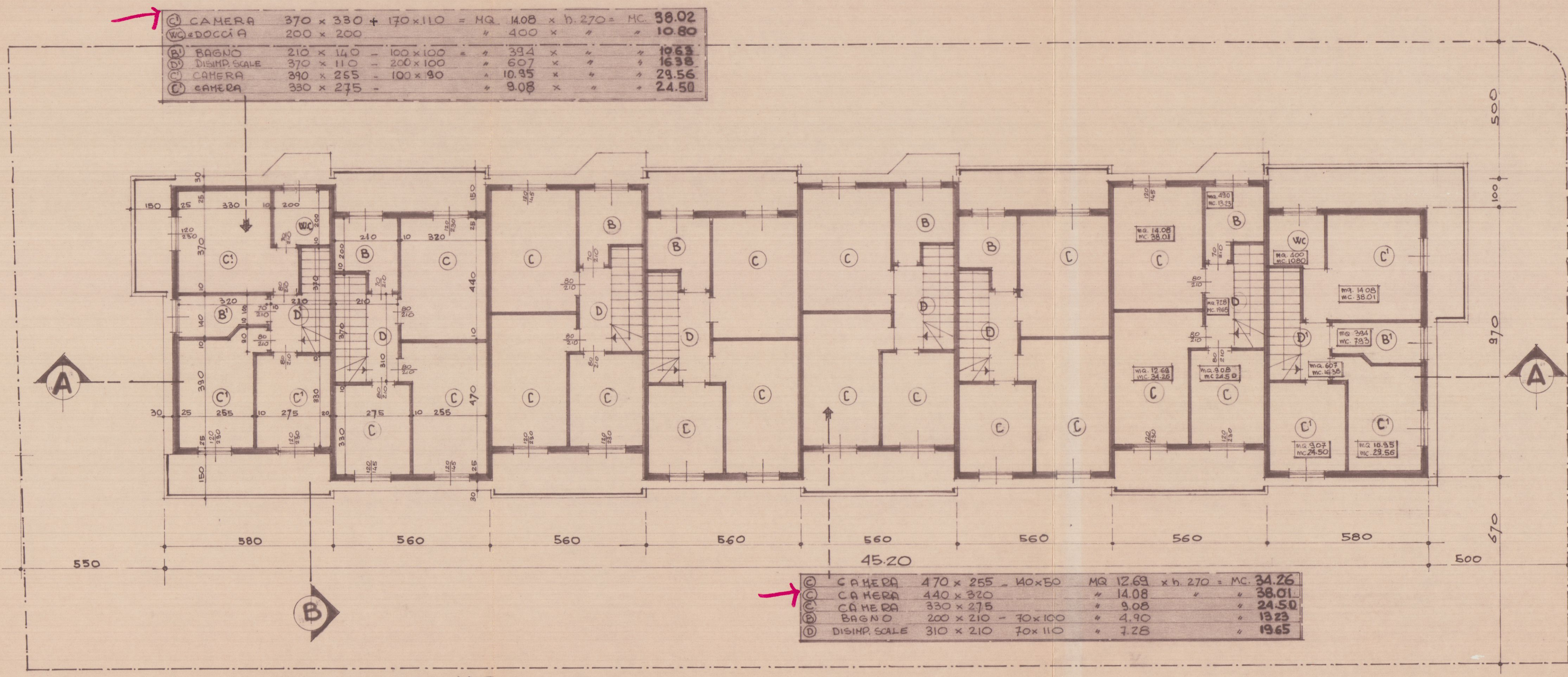
PIANO PRIMO
