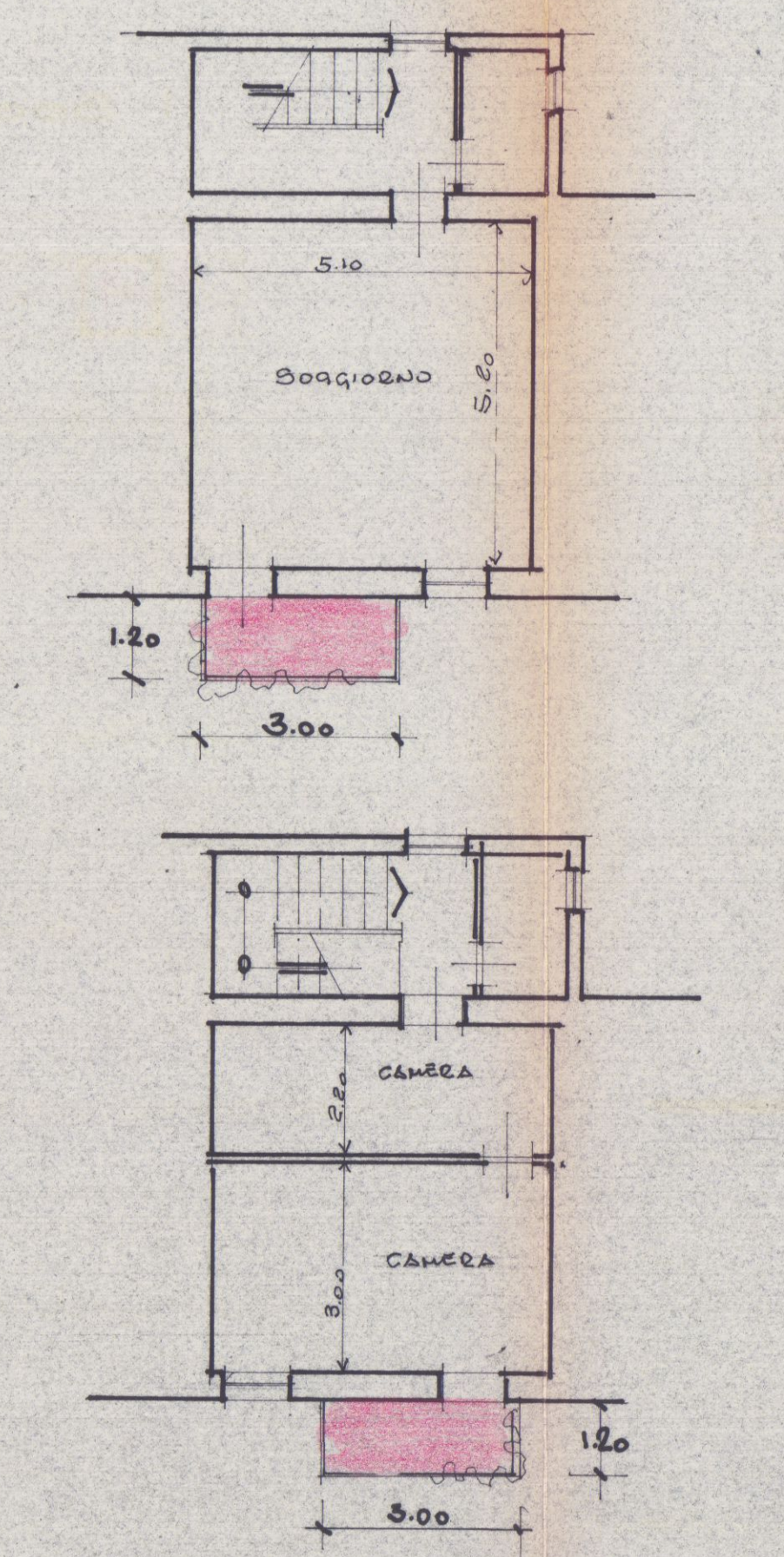
P.2° MODIFICATO
