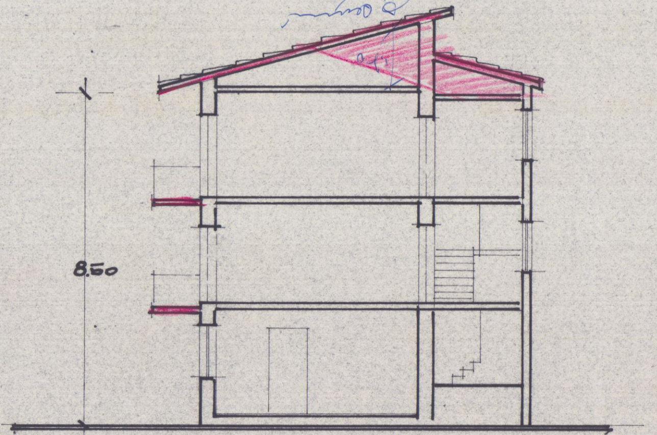
SEZIONE MODIFICATA
