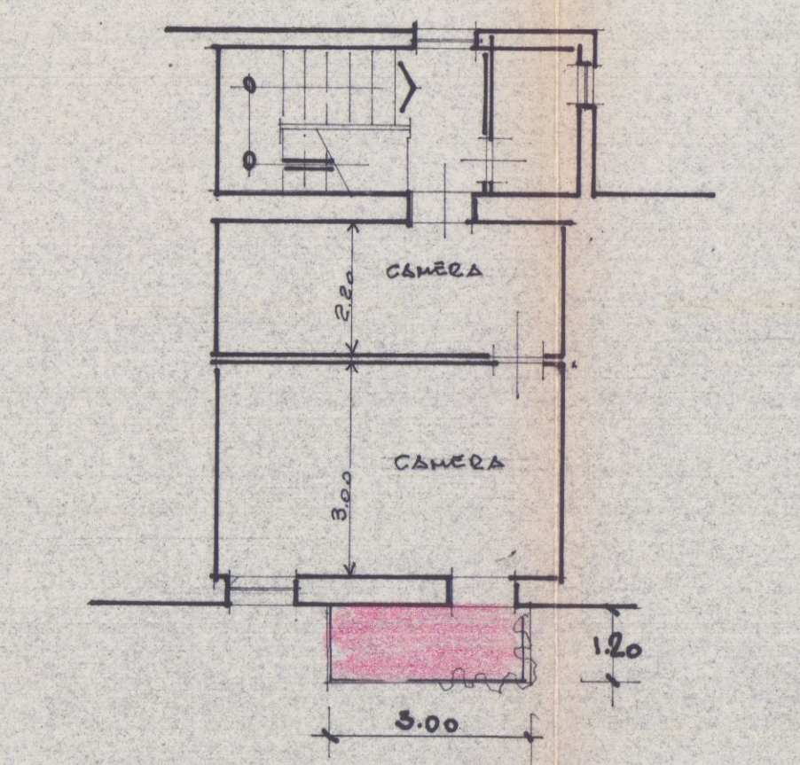
P.2° MODIFICATO
