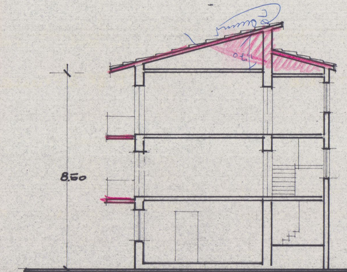
SEZIONE MODIFICATA
