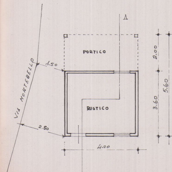
PIANTA
