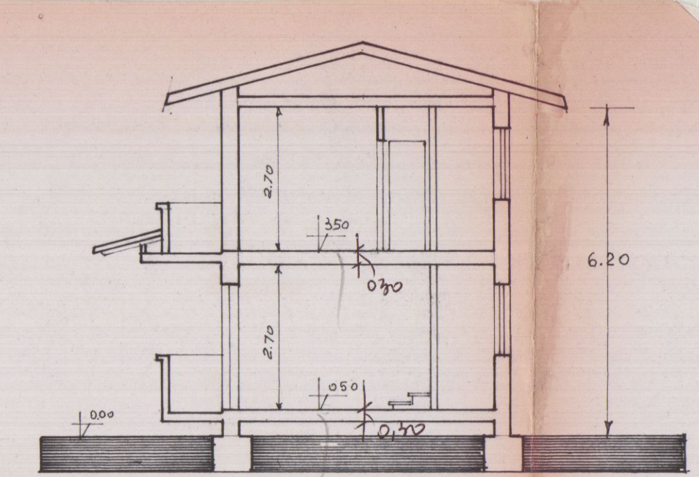
SEZIONE B-B
