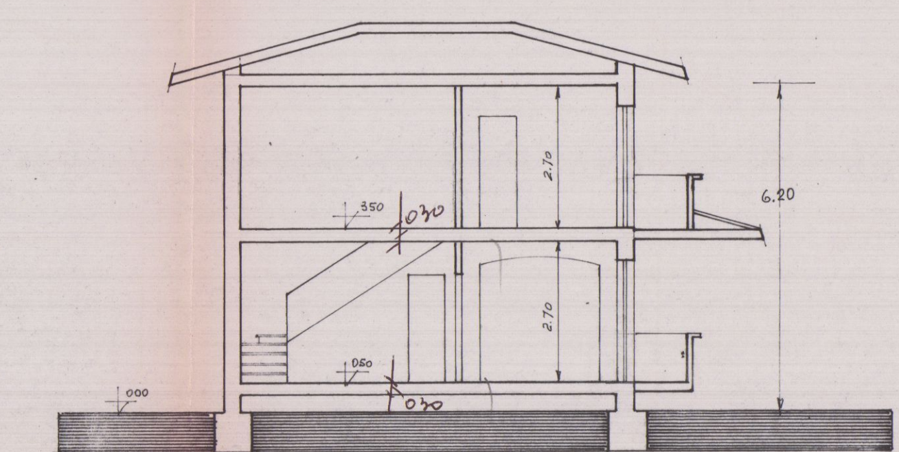
SEZIONE A-A
