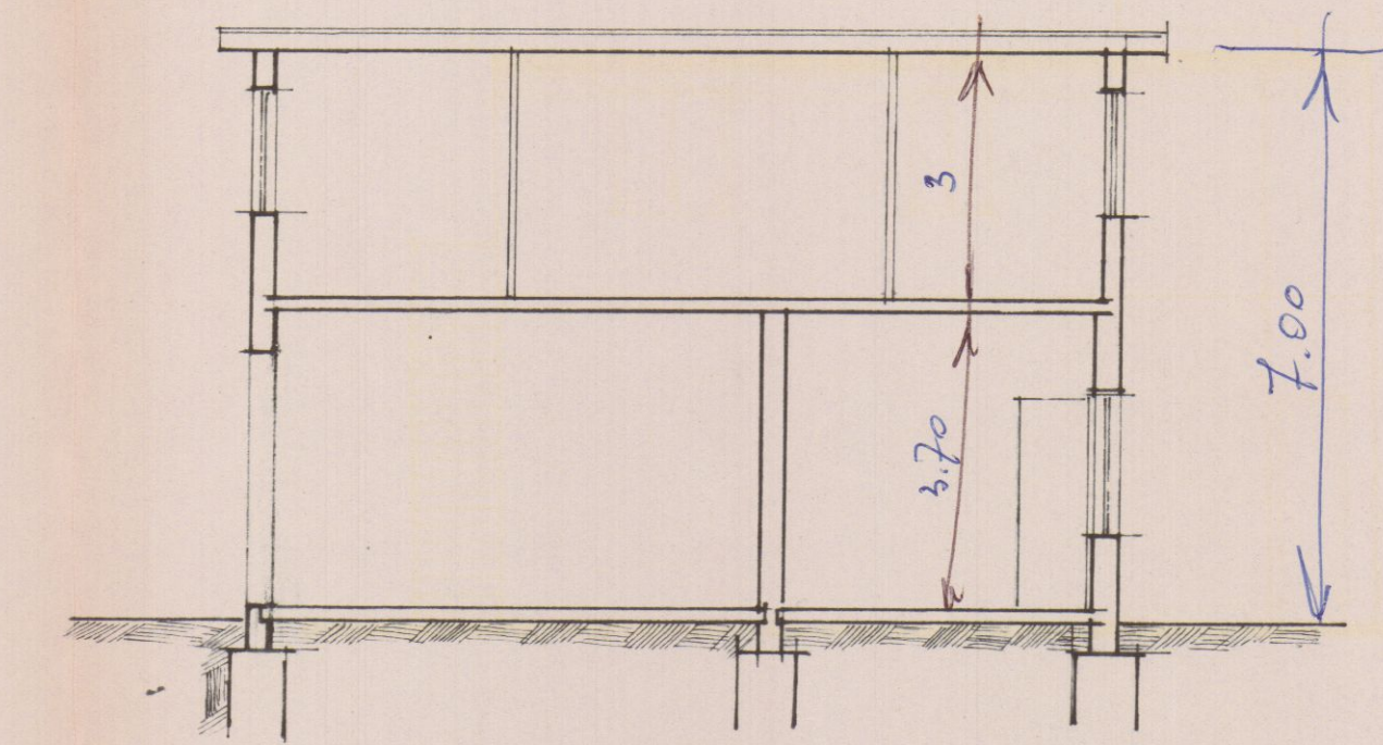
SEZIONE A - A
