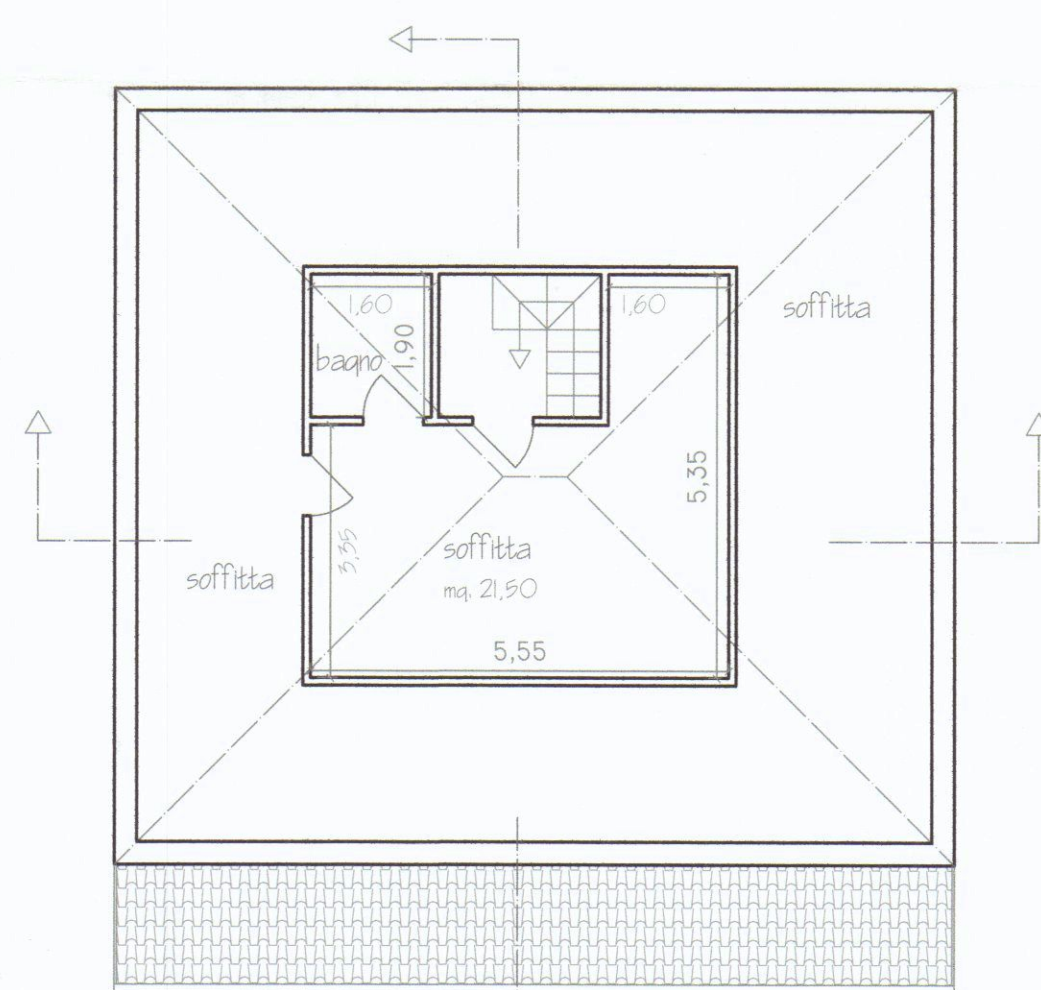
Piano Sottotetto
