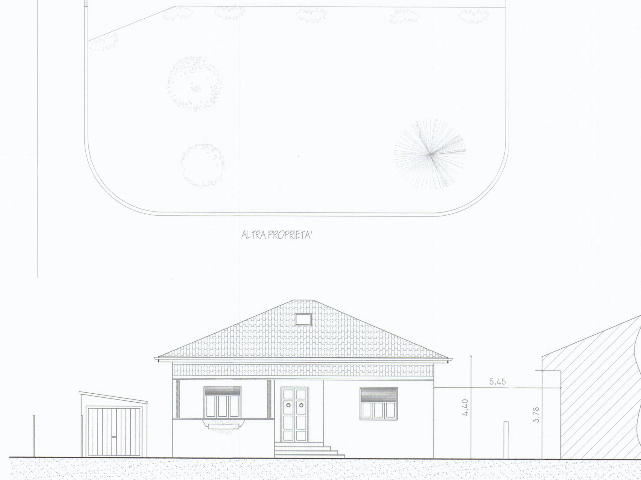
Prospetto Sud
