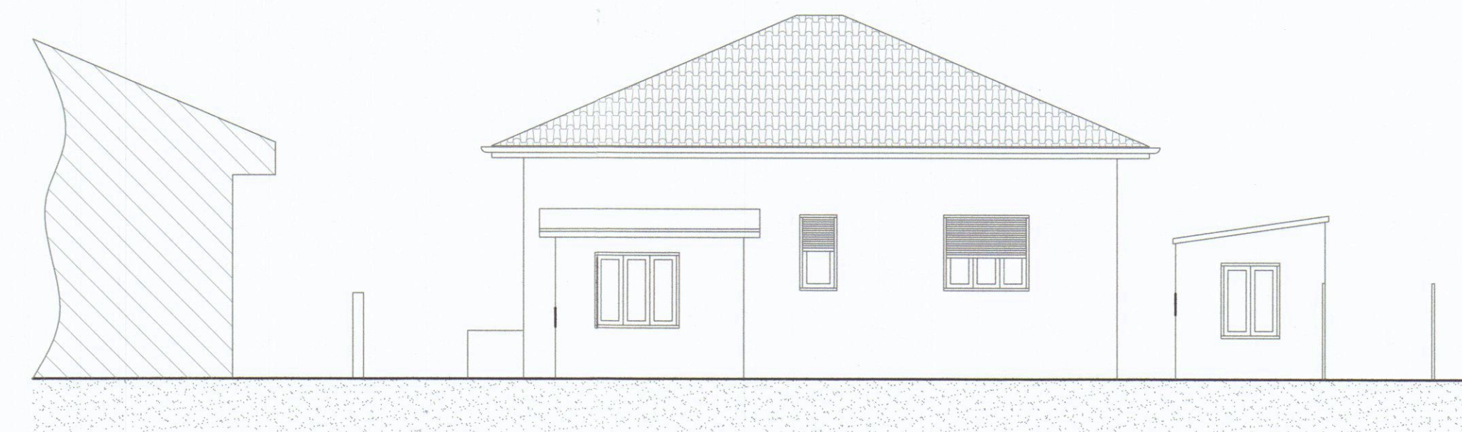
Prospetto Nord
