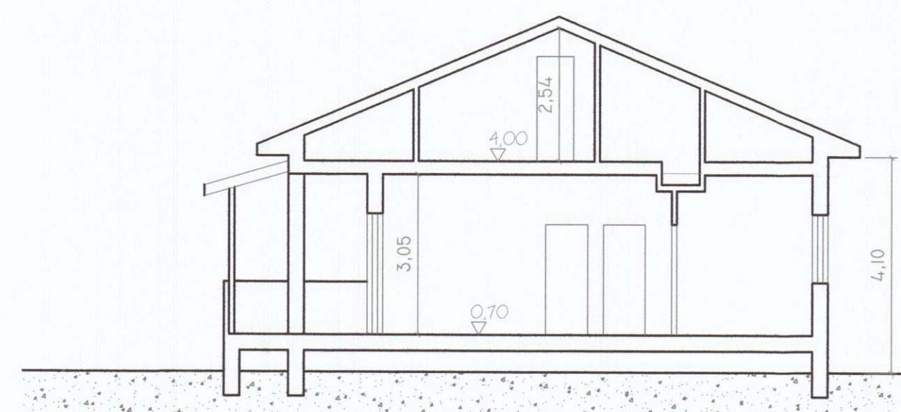
Sezione A-A'
