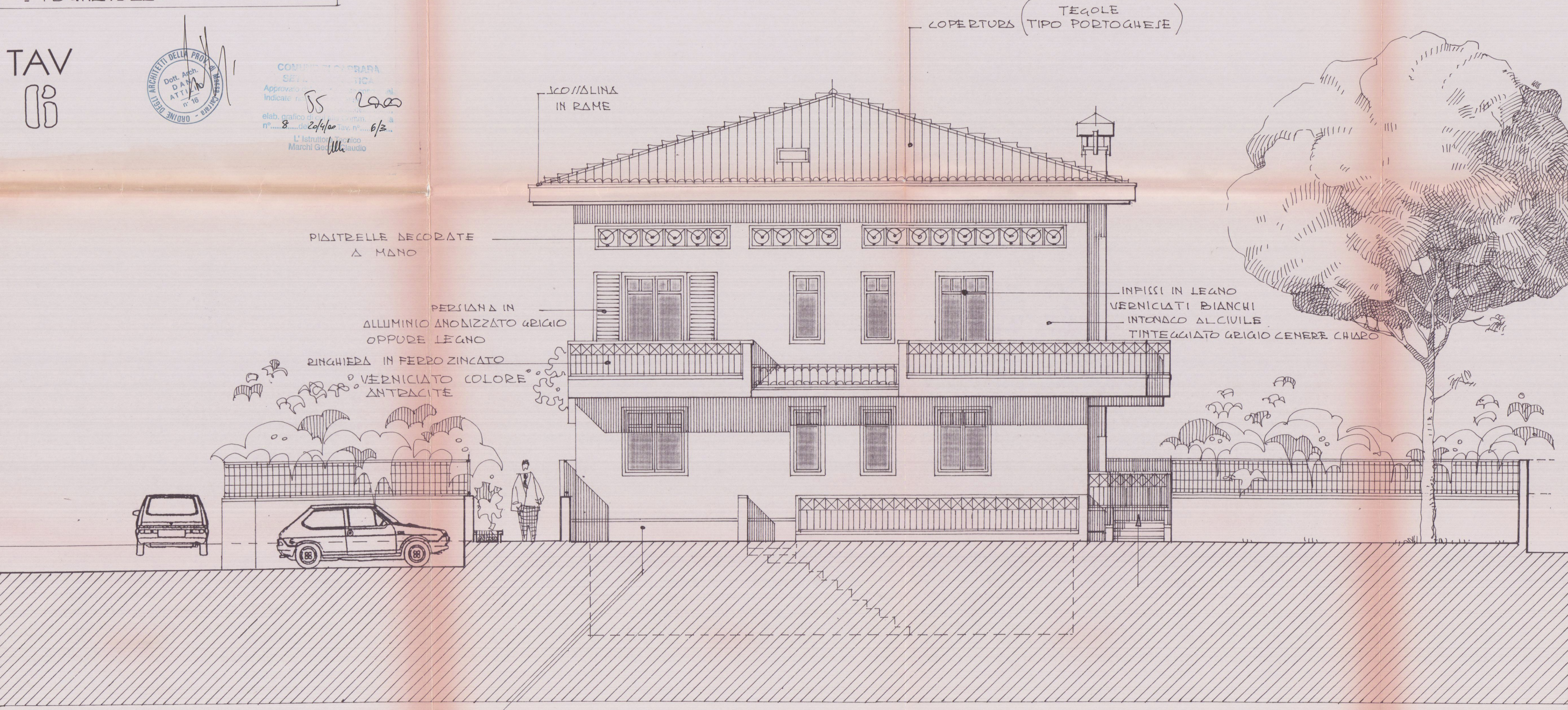
PROSPETTO OVEST
