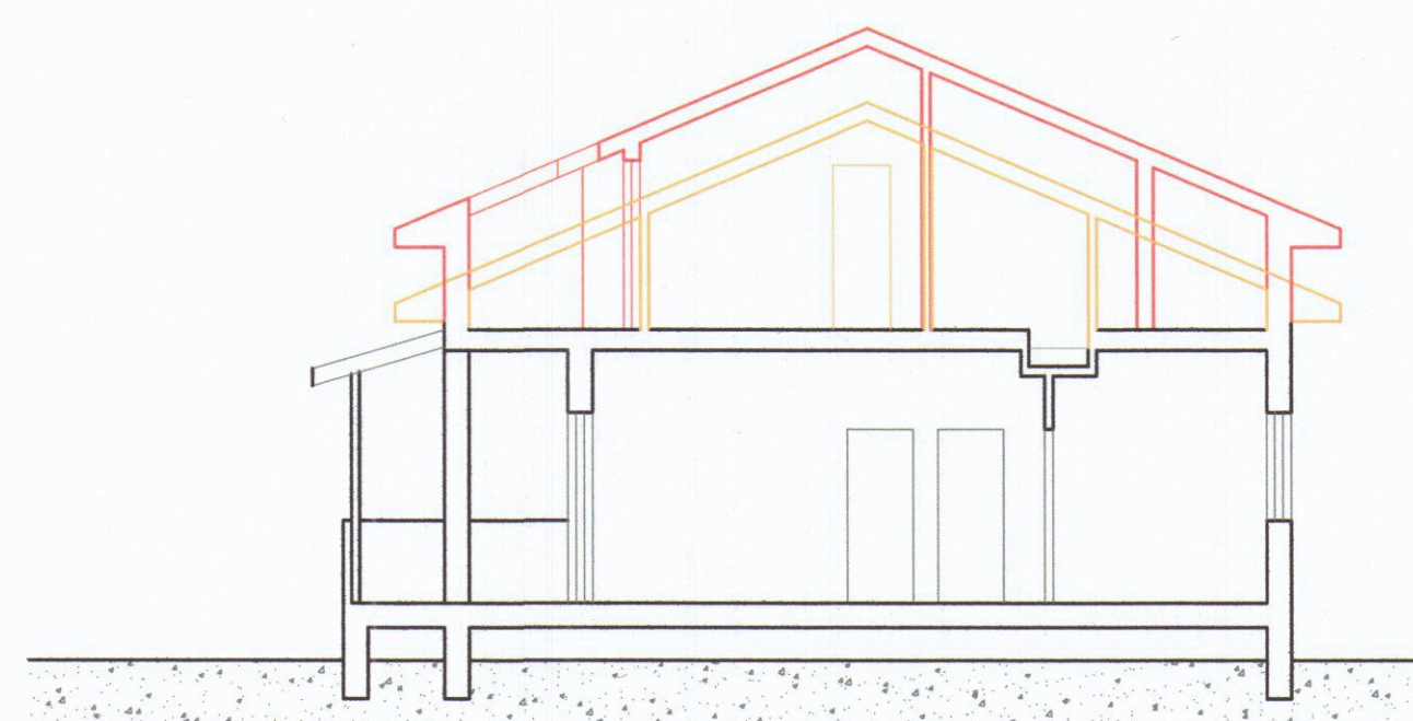
Sezione A-A'
