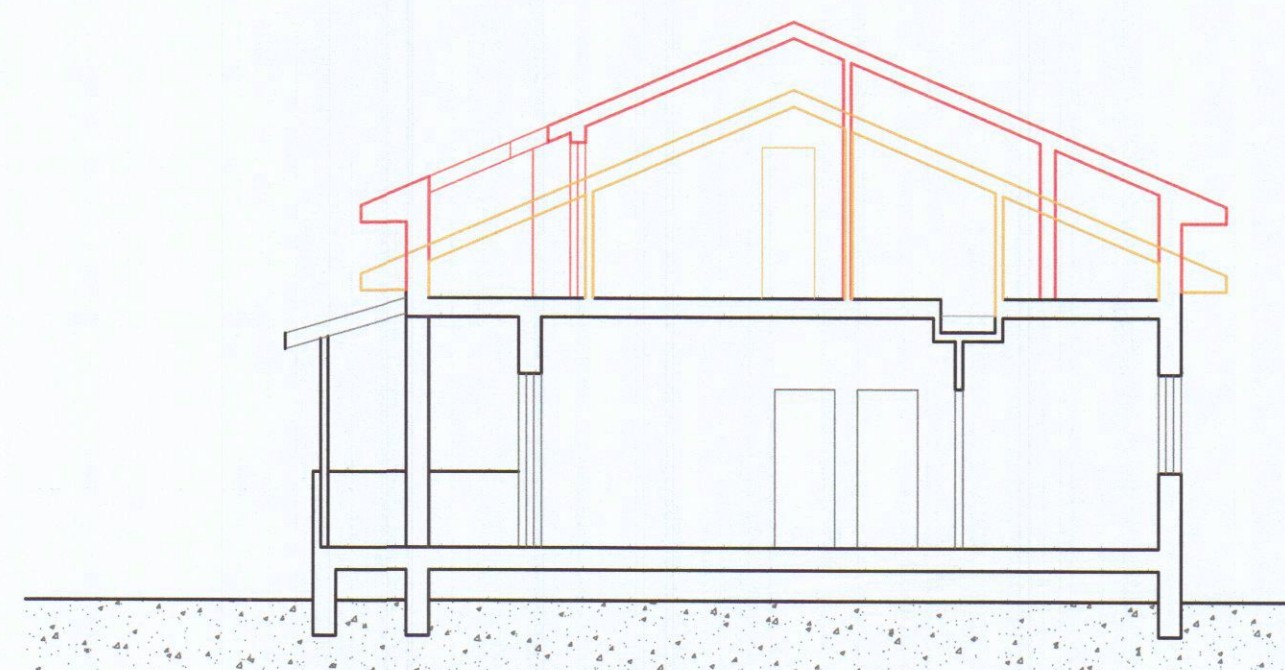
Sezione A-A'
