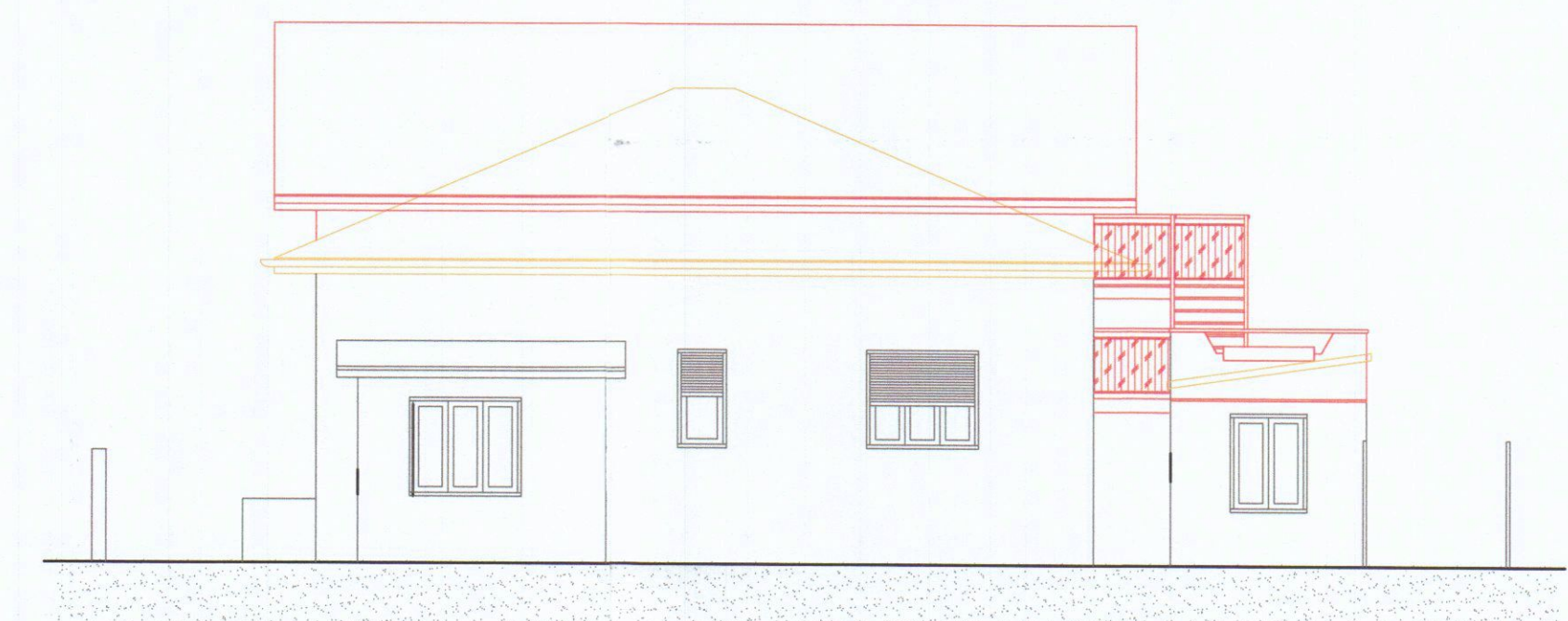
Prospetto Nord
