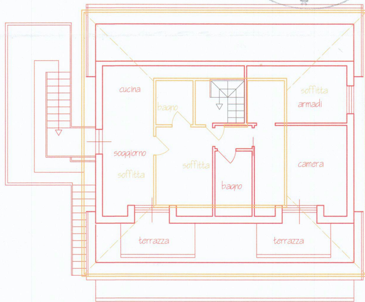
Piano Sottotetto
