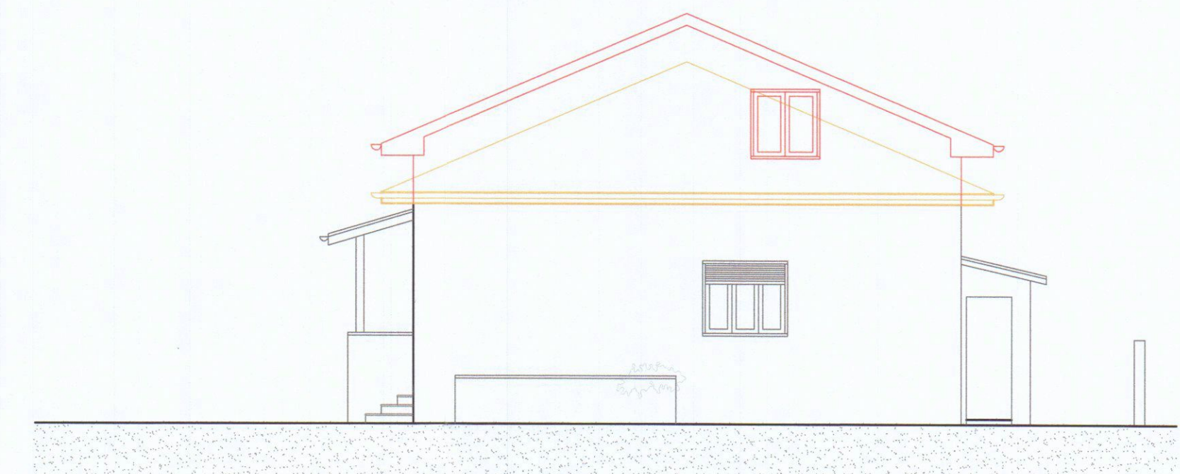
Prospetto Est
