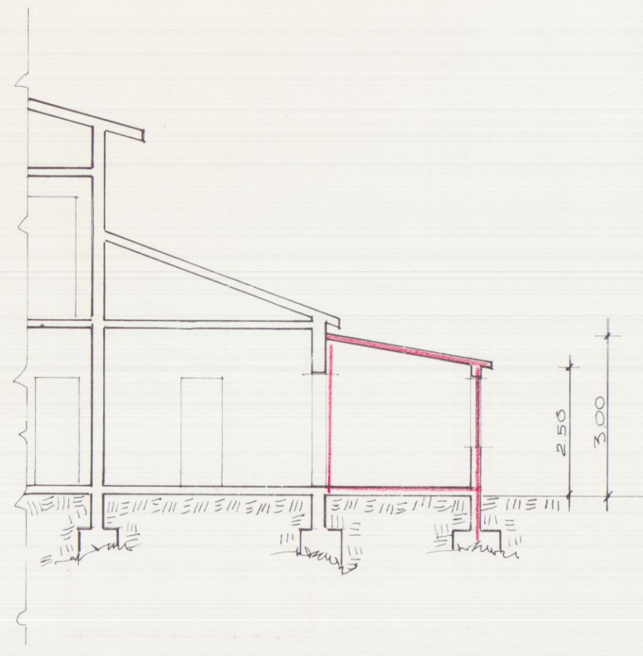
SEZIONE A-A
