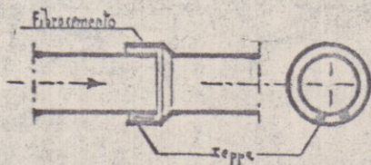
SUB-IRRIGAZIONE SEMPLICE CON FINALE A DOZZO PERDENTE
