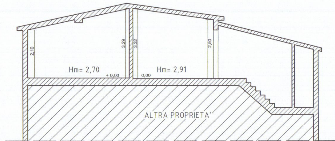
SEZIONE A-A STATO ATTUALE
