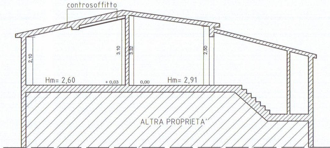
SEZIONE A-A STATO PROGETTO
