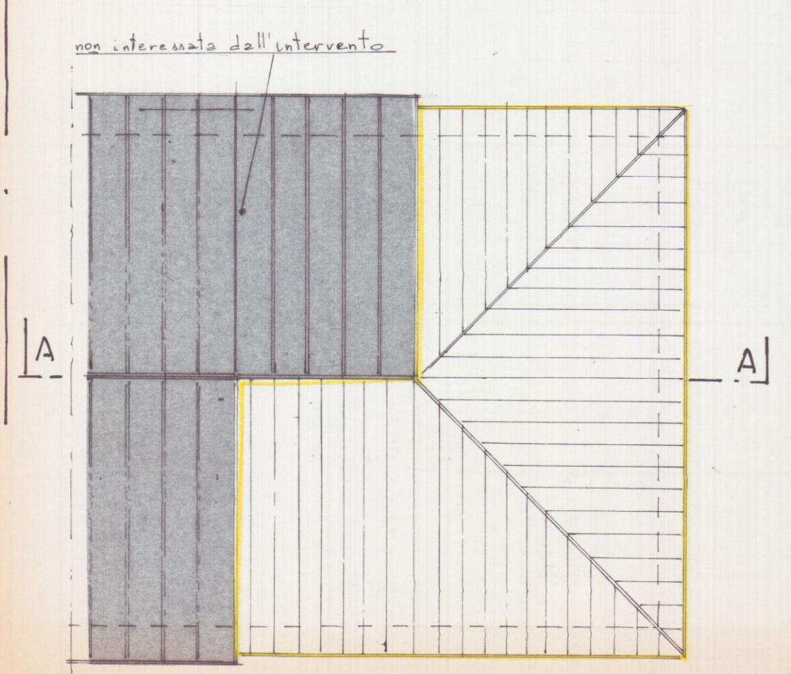
COPERTURA
