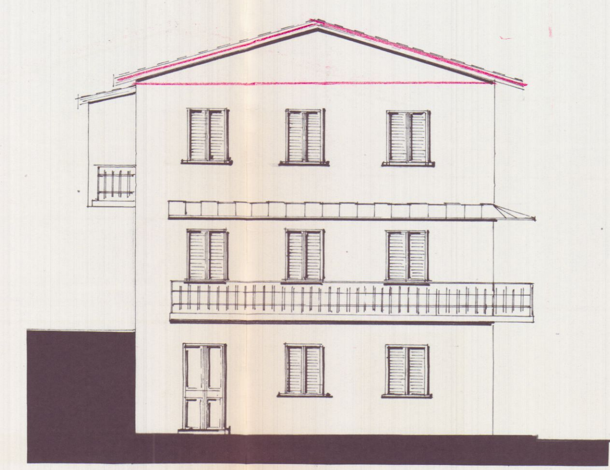
PROSPETTO SUD
