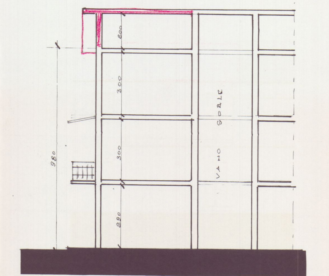
SEZIONE A-A
