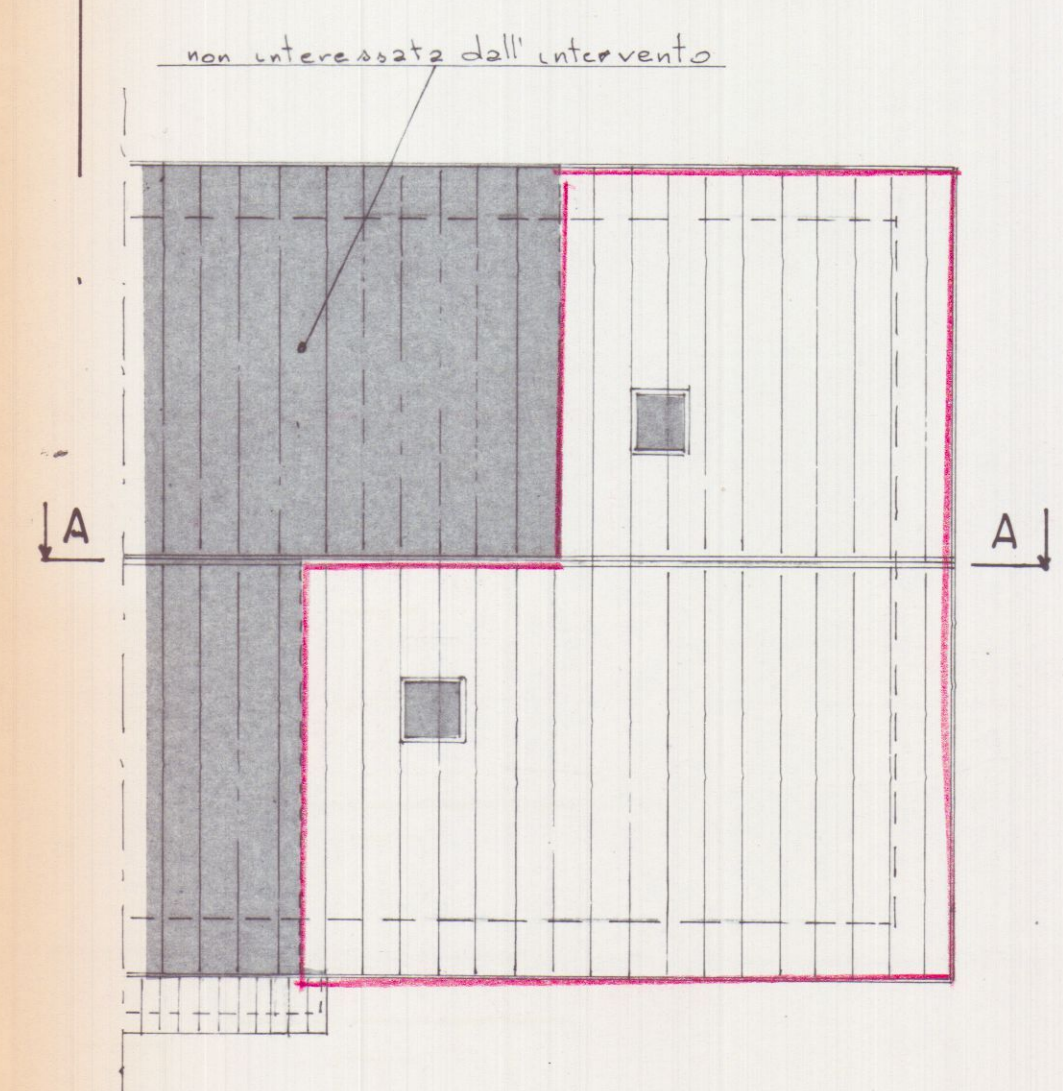
COPERTURA
