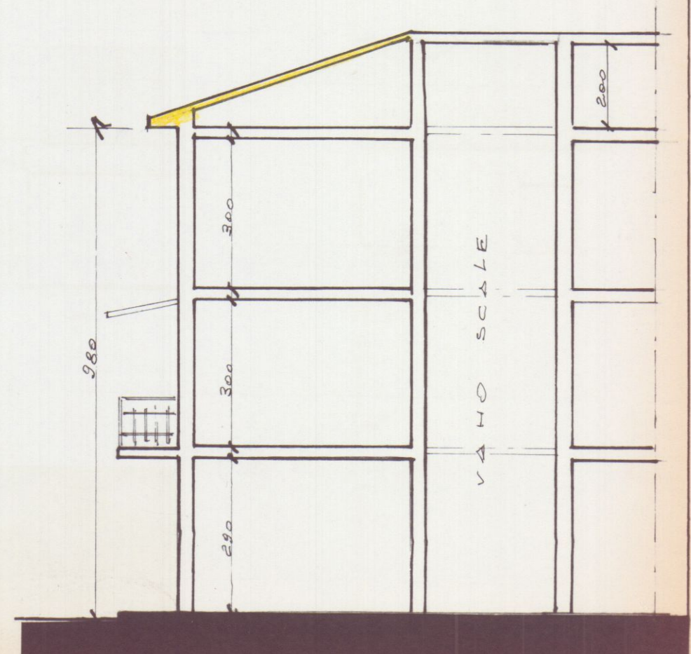
SEZIONE A-A
