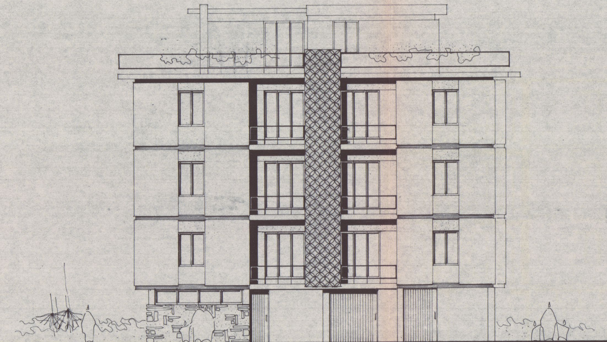
- PROSPETTO SUD -
