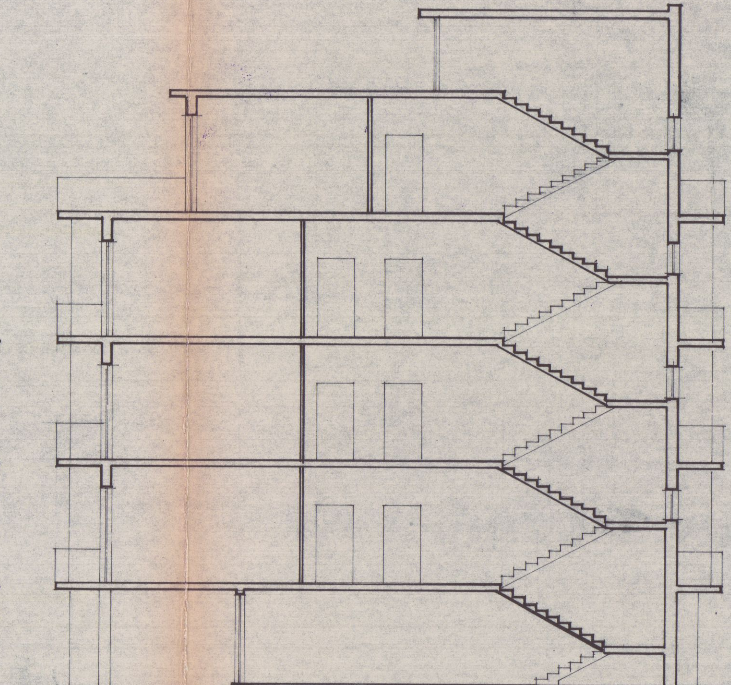
- SEZIONE -
