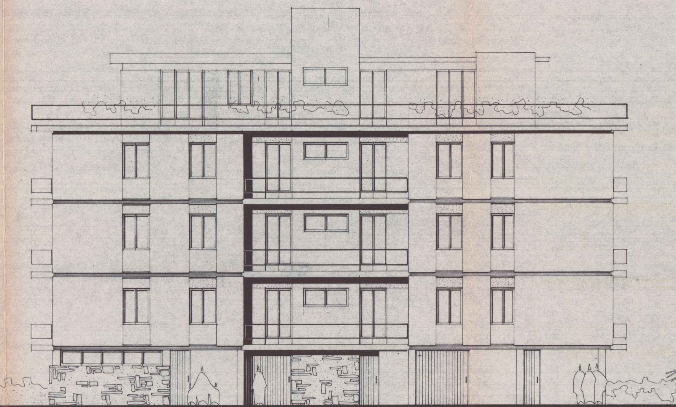
- PROSPETTO OVEST -
