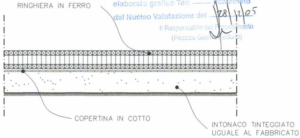
PARTICOLARE RECINZIONE
