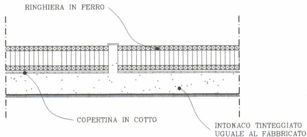
PARTICOLARE RECINZIONE
