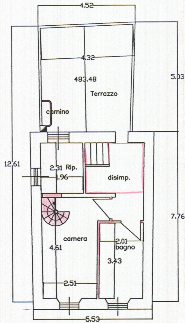
Pianta Piano Terzo
