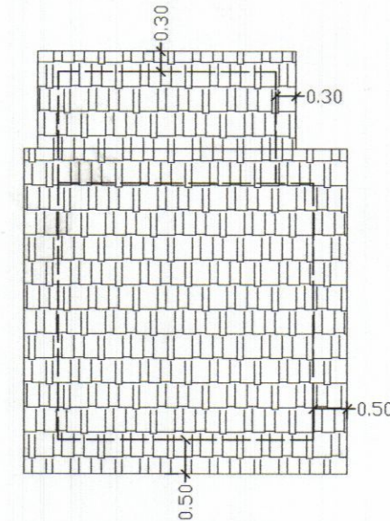
PIANTA COPERTURA
