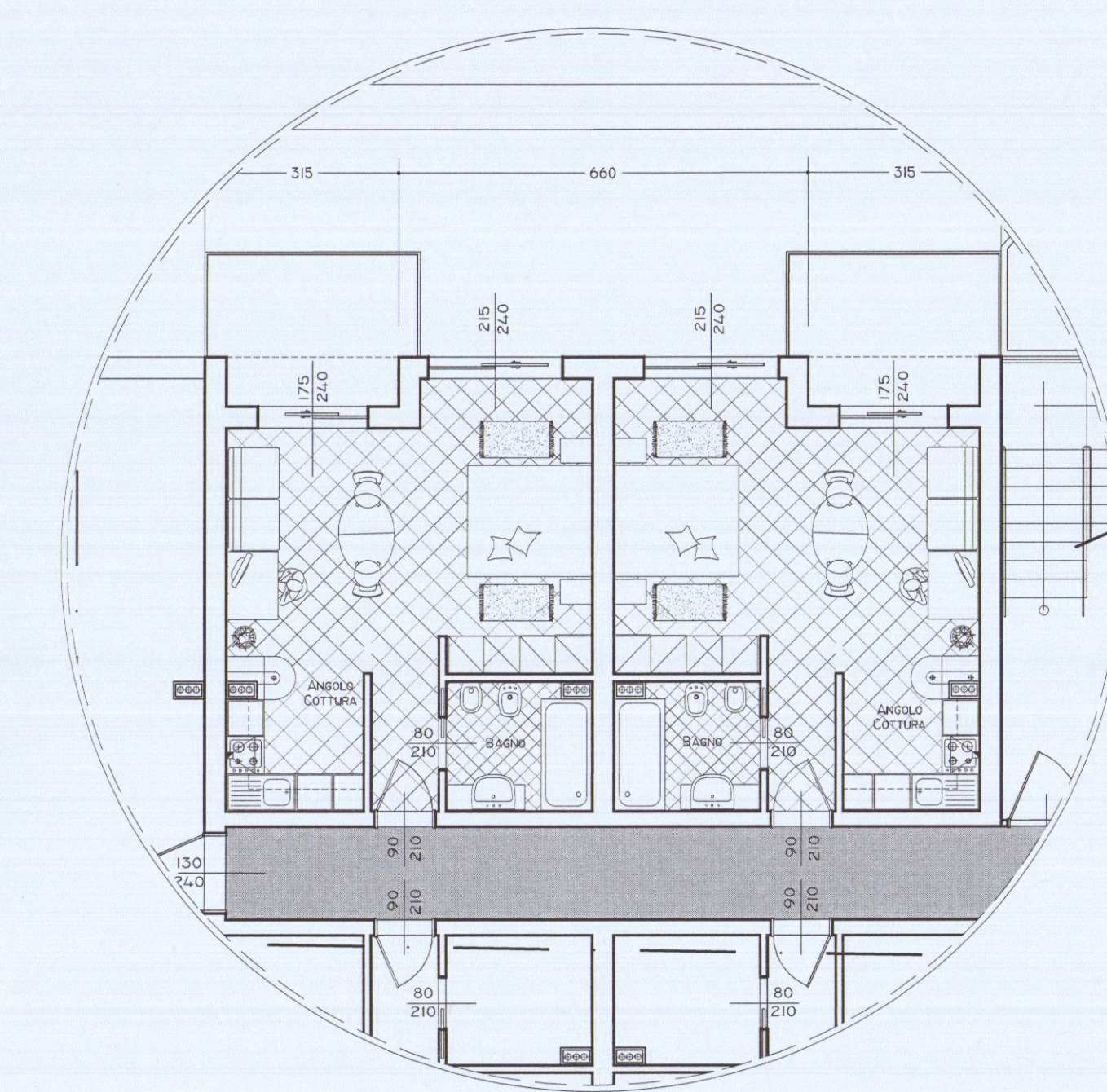
PLANIMETRIE CAMERE TIPO - ARREDO CAMERE 37-38
