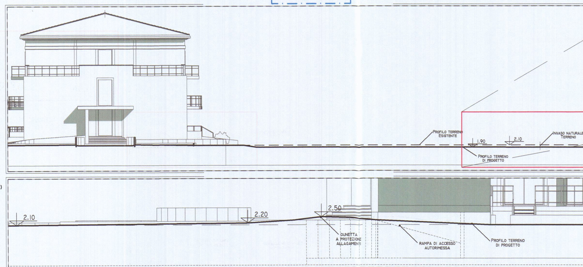
PARTICOLARE 3 (SEZIONE B) SCALA 1:100 MODELLAZIONE MIRATA TERRENO PROFONDITÀ MT. 0.20/0.25 MC. 140 (L'INTERVENTO È PREVISTO SU AMBEDUE LE RAMPE)
