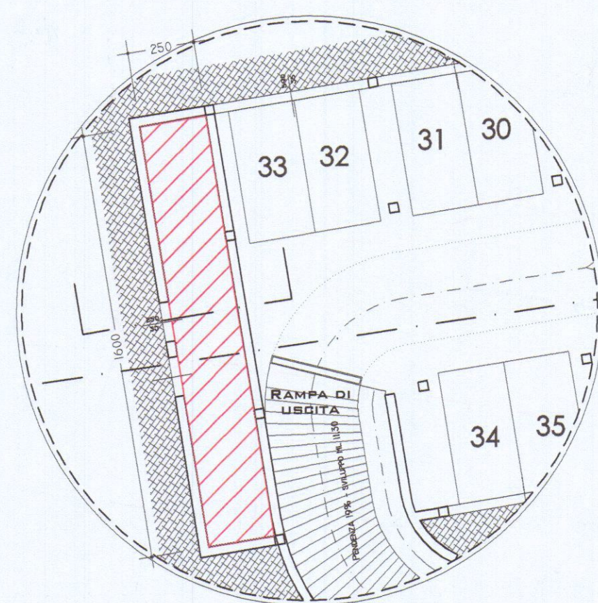
PARTICOLARE 1 VASCA DI RACCOLTA PRIMA PIOGGIA MC. 43
