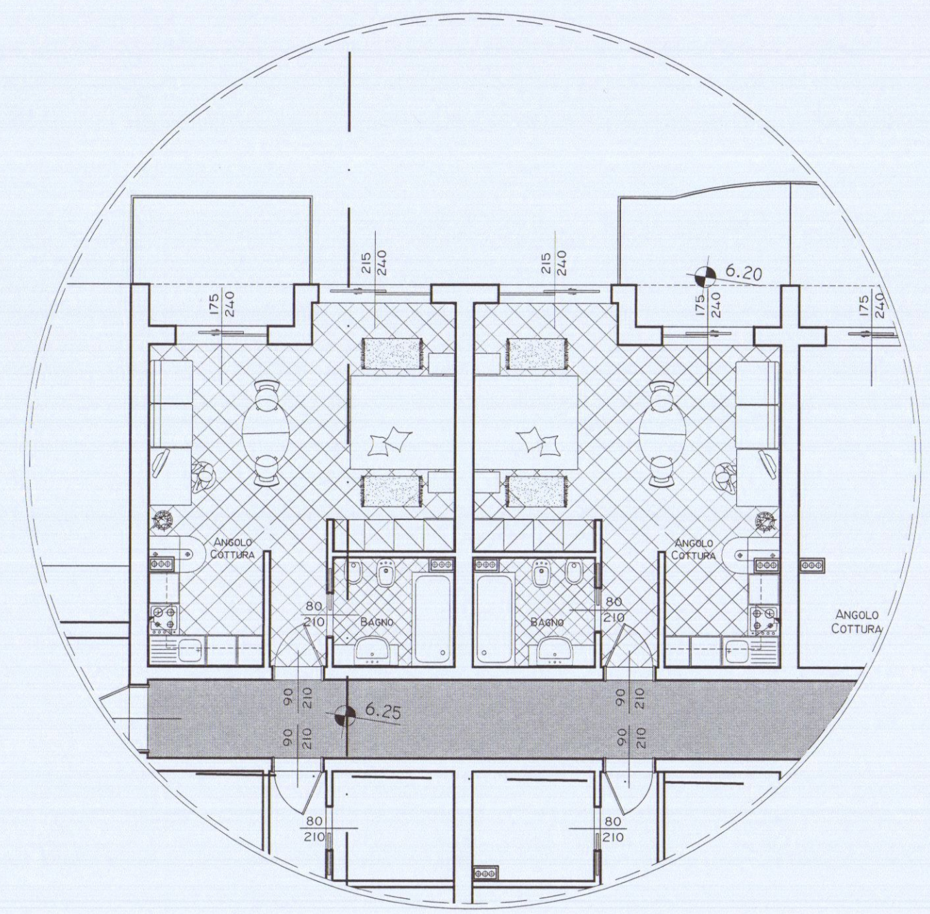
PLANIMETRIE CAMERE TIPO - ARREDO CAMERE 19-20
