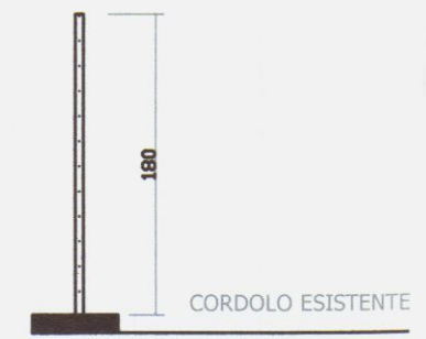
SEZIONE TIPO SCALA 1:50
